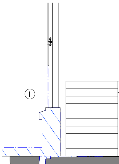
5 Section BB Scale: 1:50
