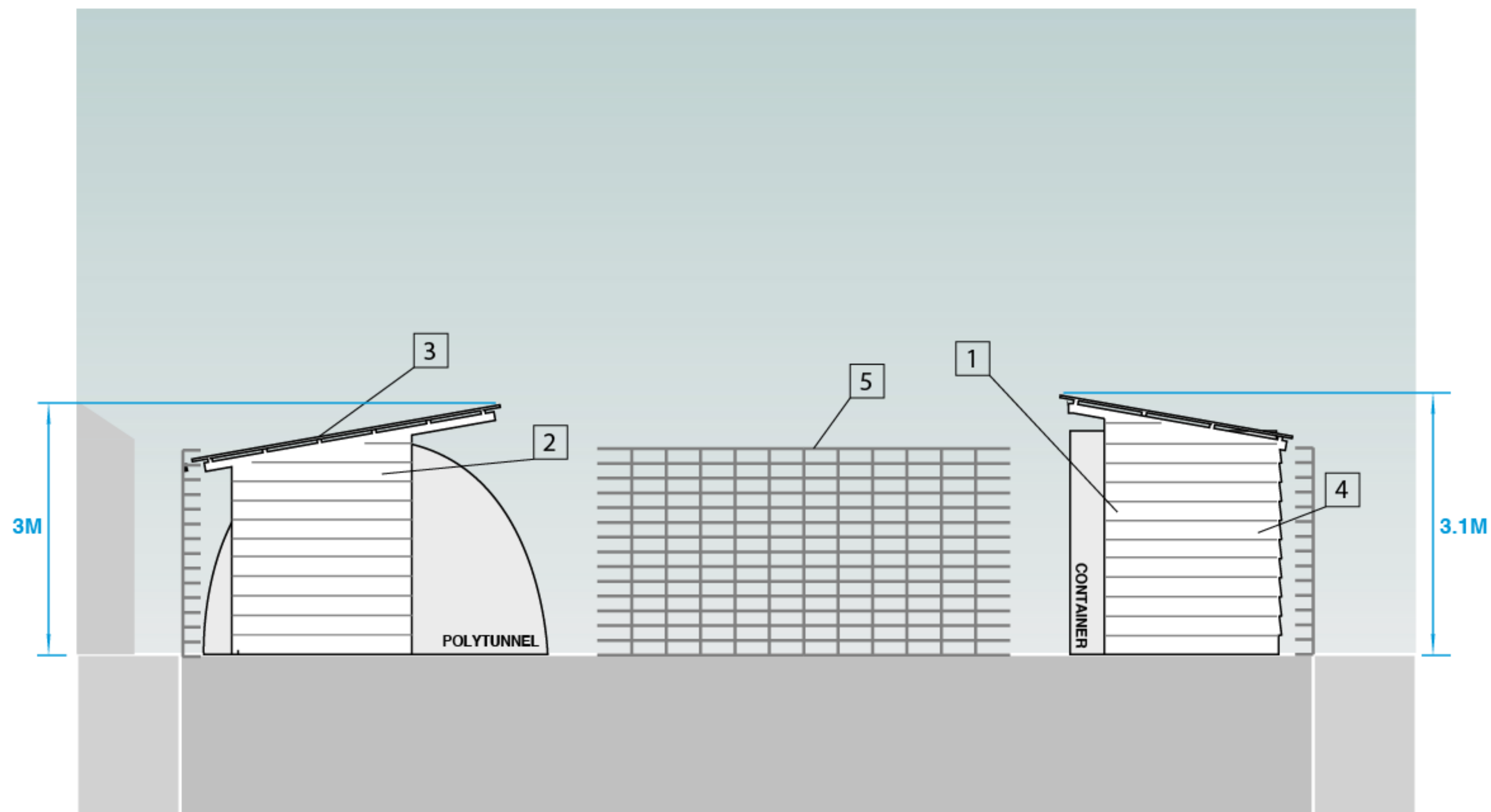
Elevation 1
