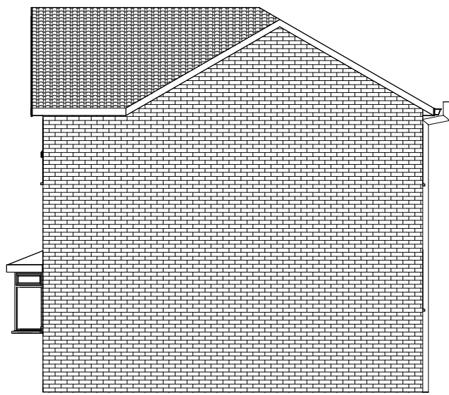
Existing Side 1 : 100
