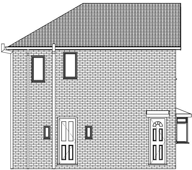
Existing Side (2) 1 : 100
