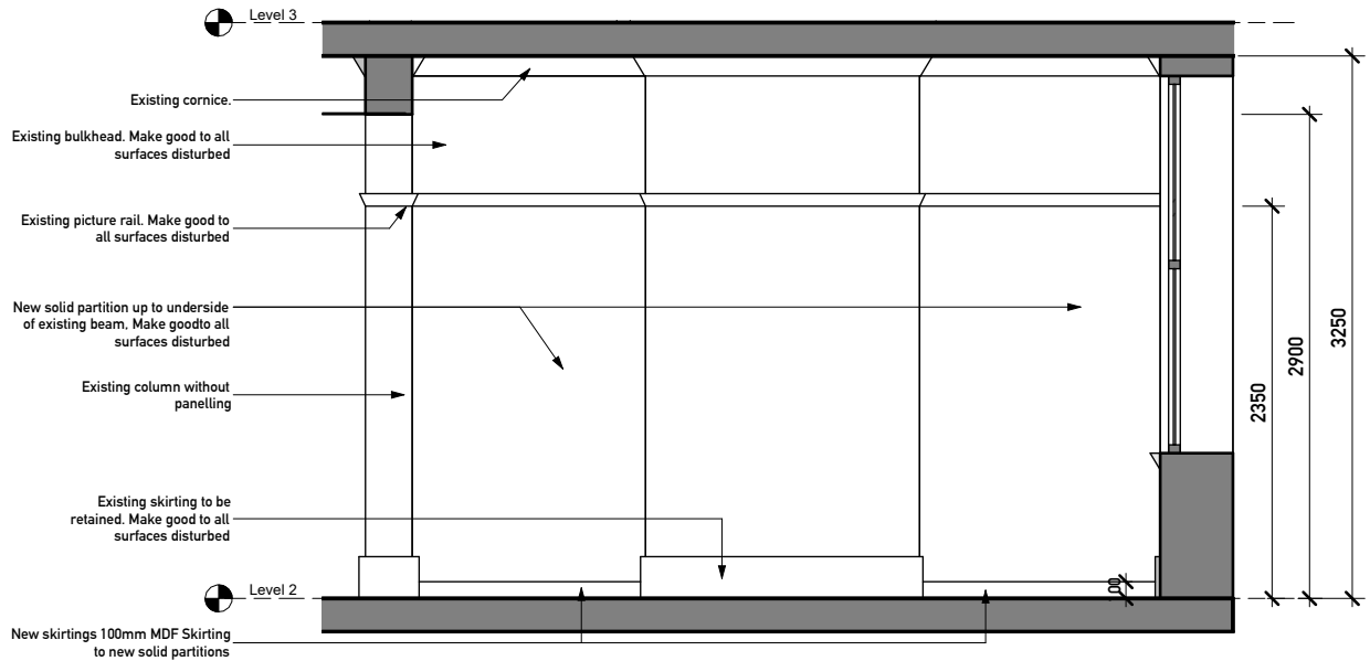
4 L2 Section 4 02-500 1 : 50
