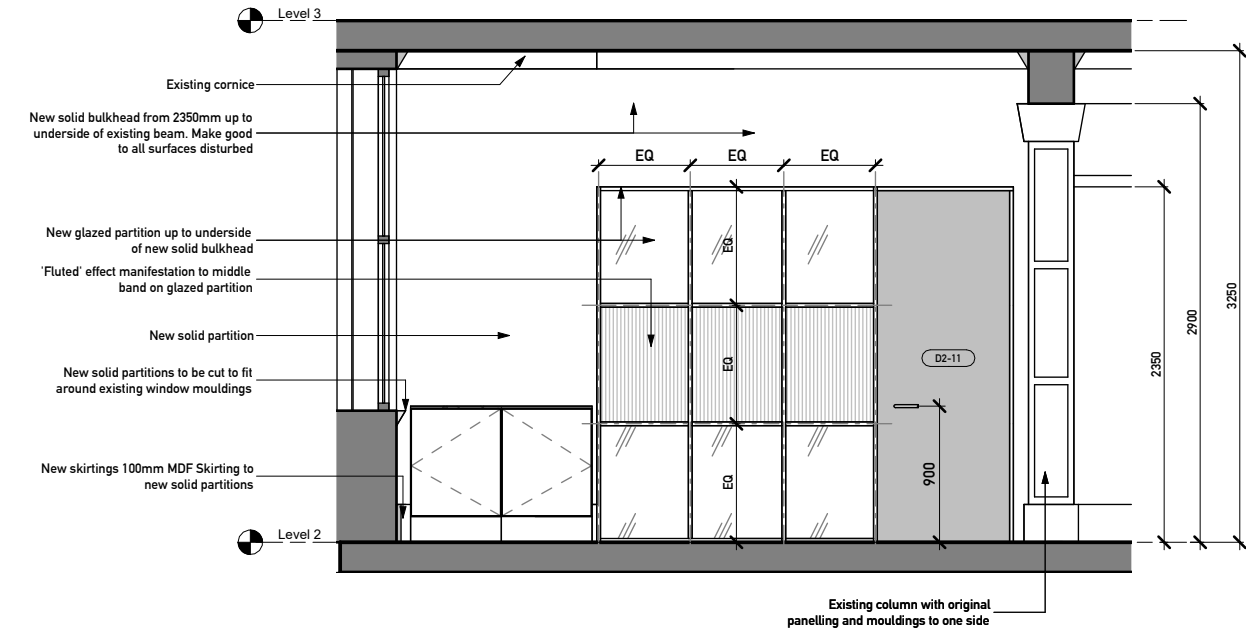
3 L2 Section 3 02-500 1 : 50
