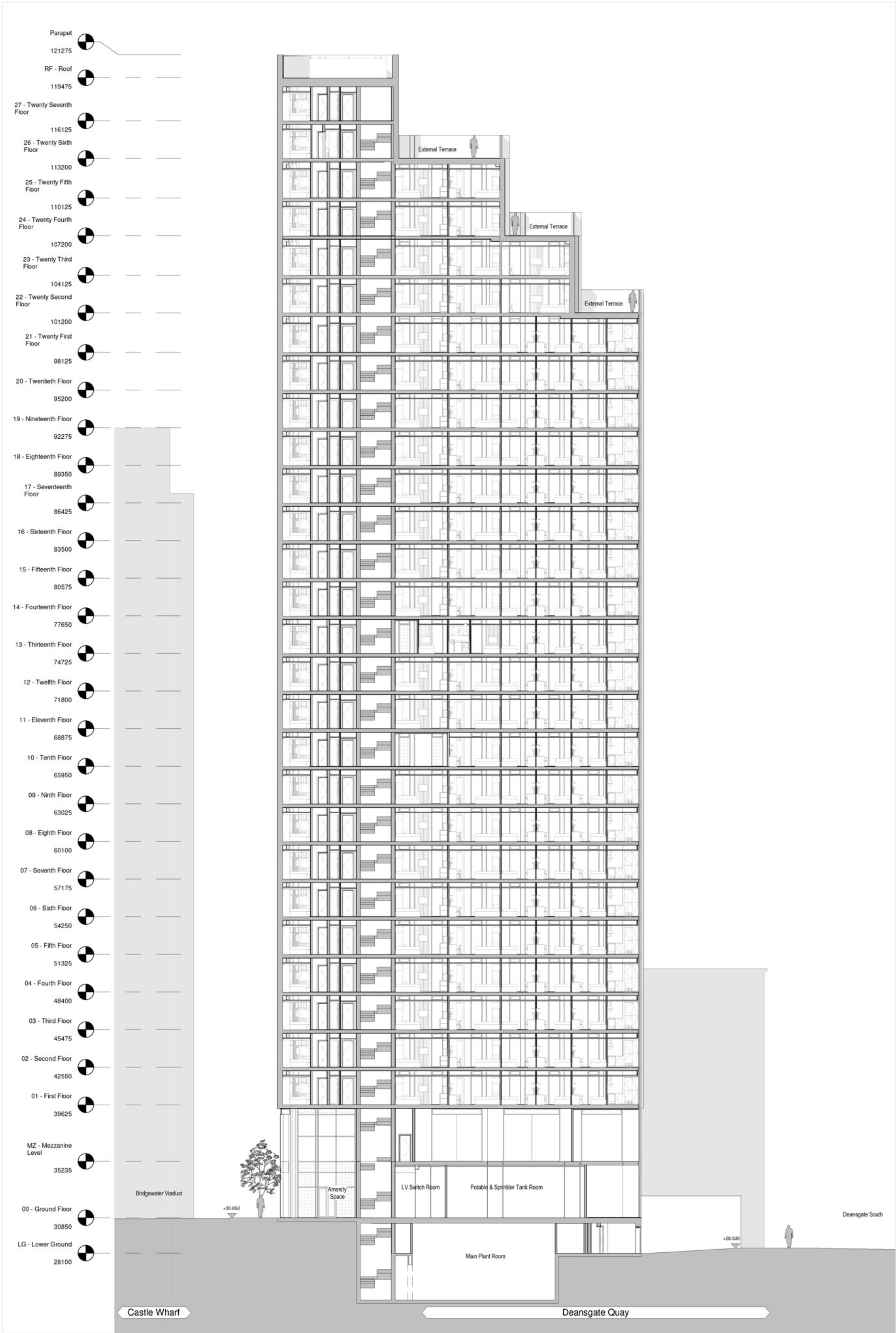
01 Section C-C 1 : 200
