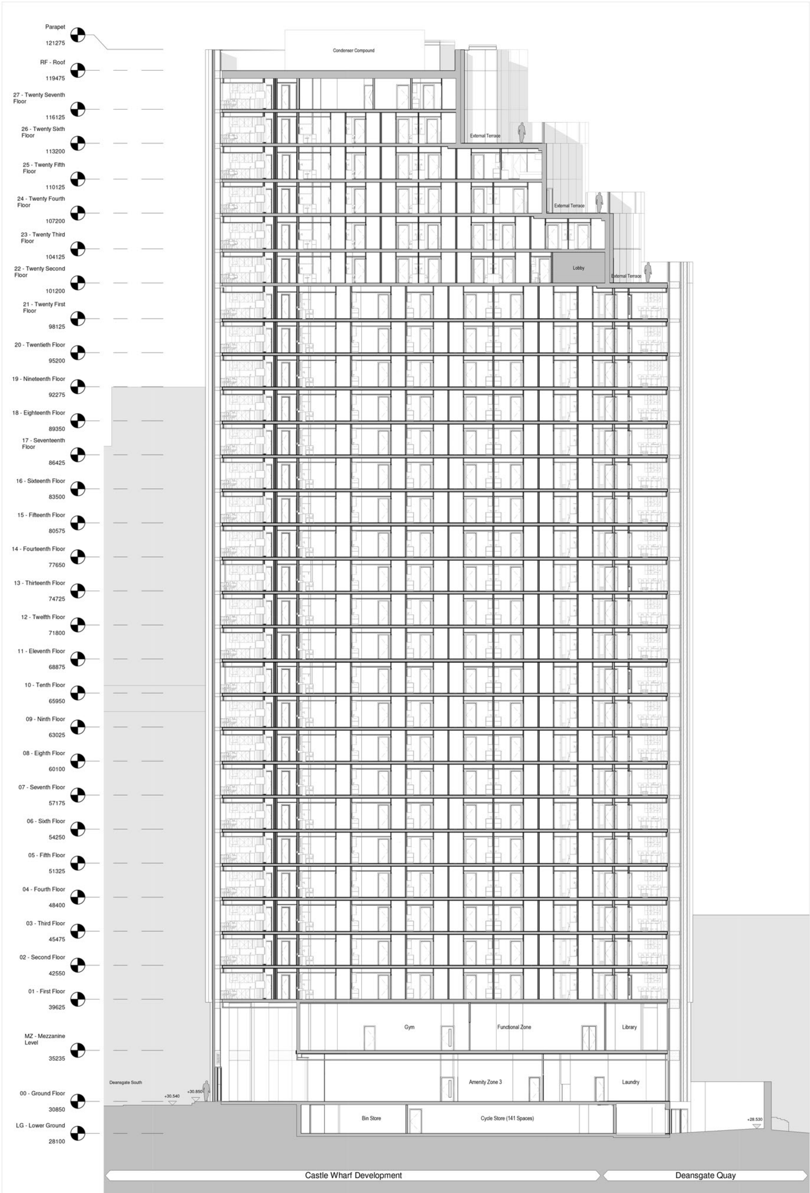
01 Section A-A 1 : 200
