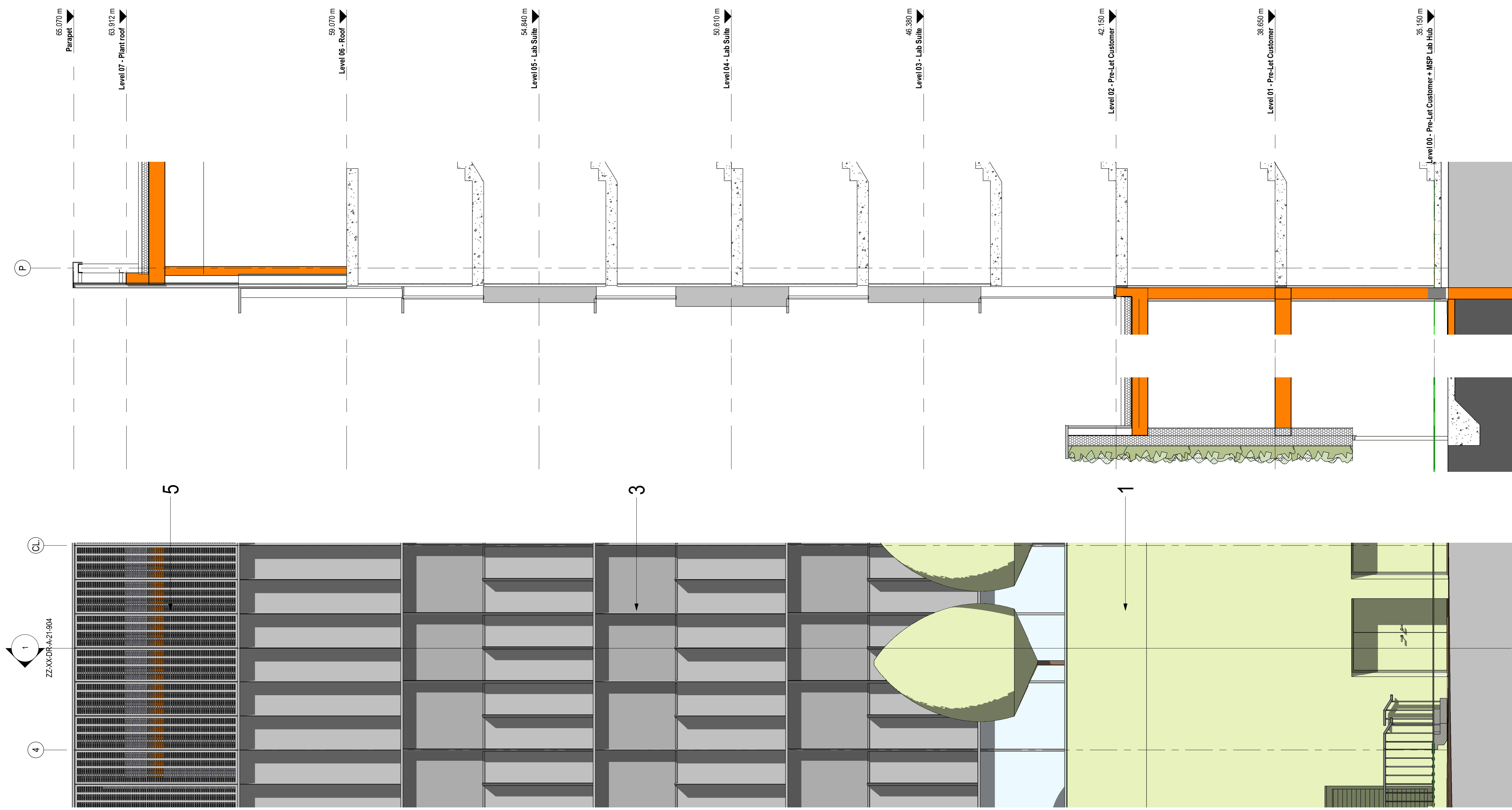
Elevation 1:50
