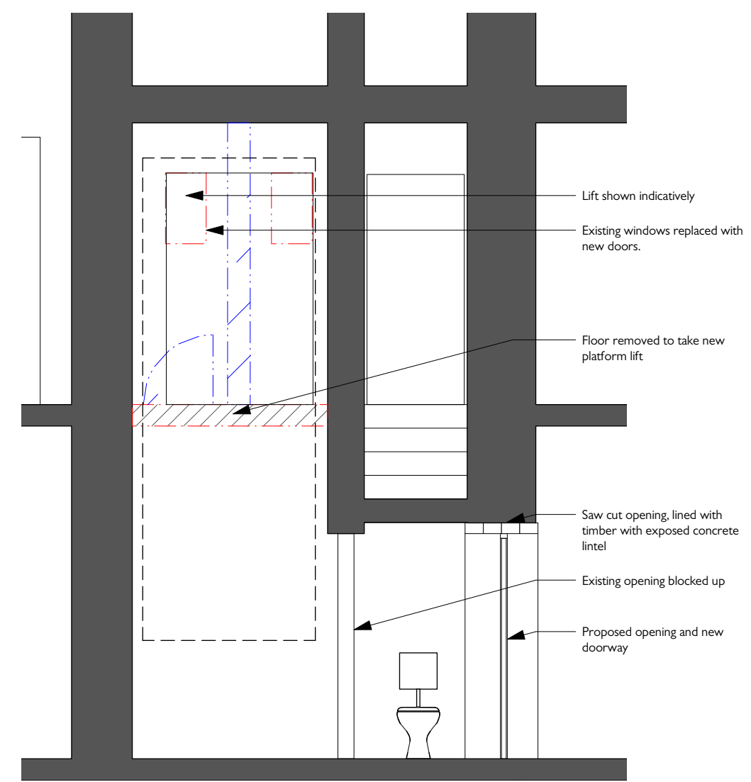
I Section GG Scale: 1:50
