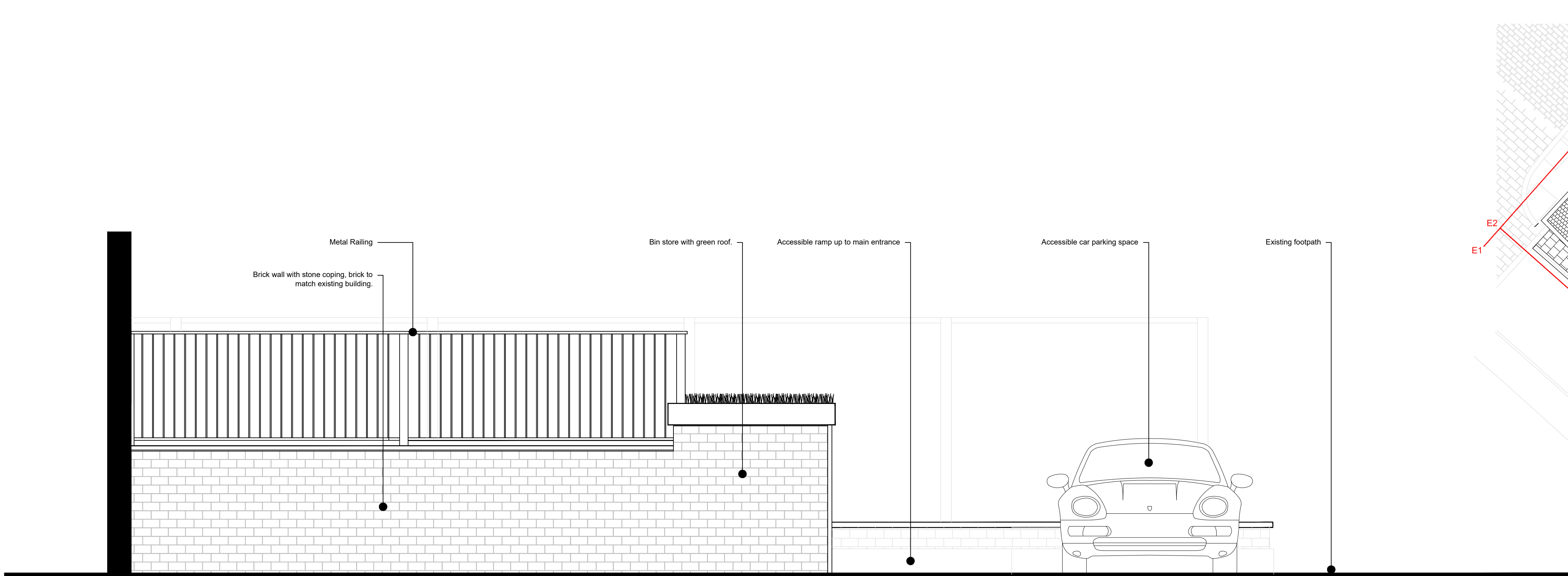
Elevation E1 - E1' - Blossom Street
