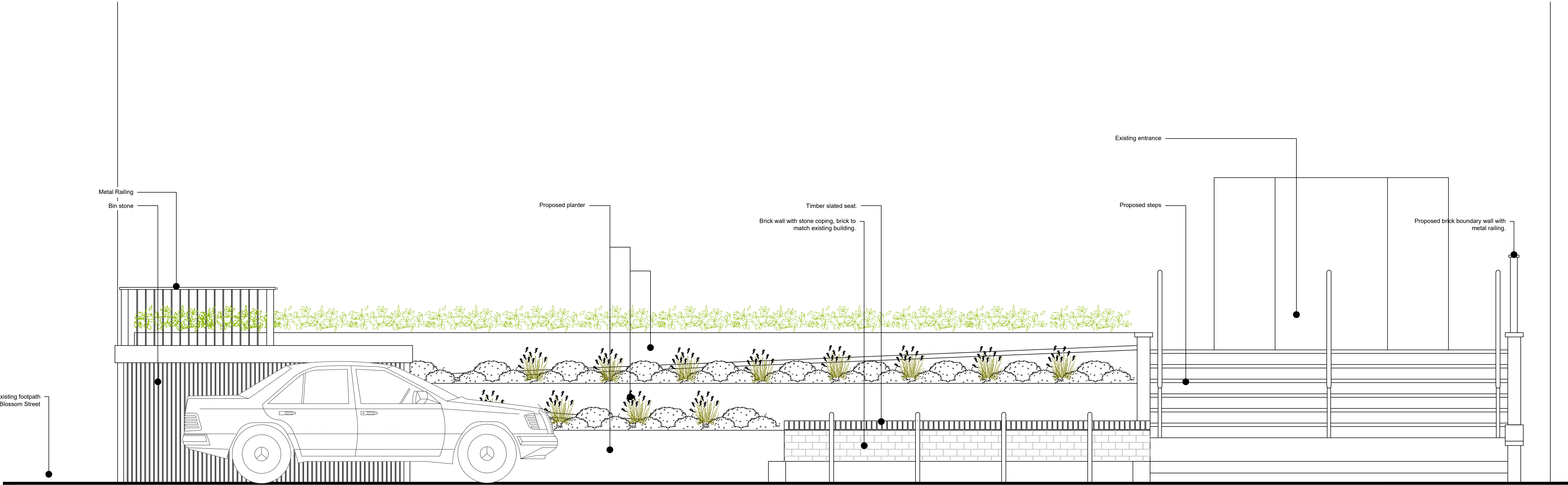
Elevation E2 - E2' - Gun Street
