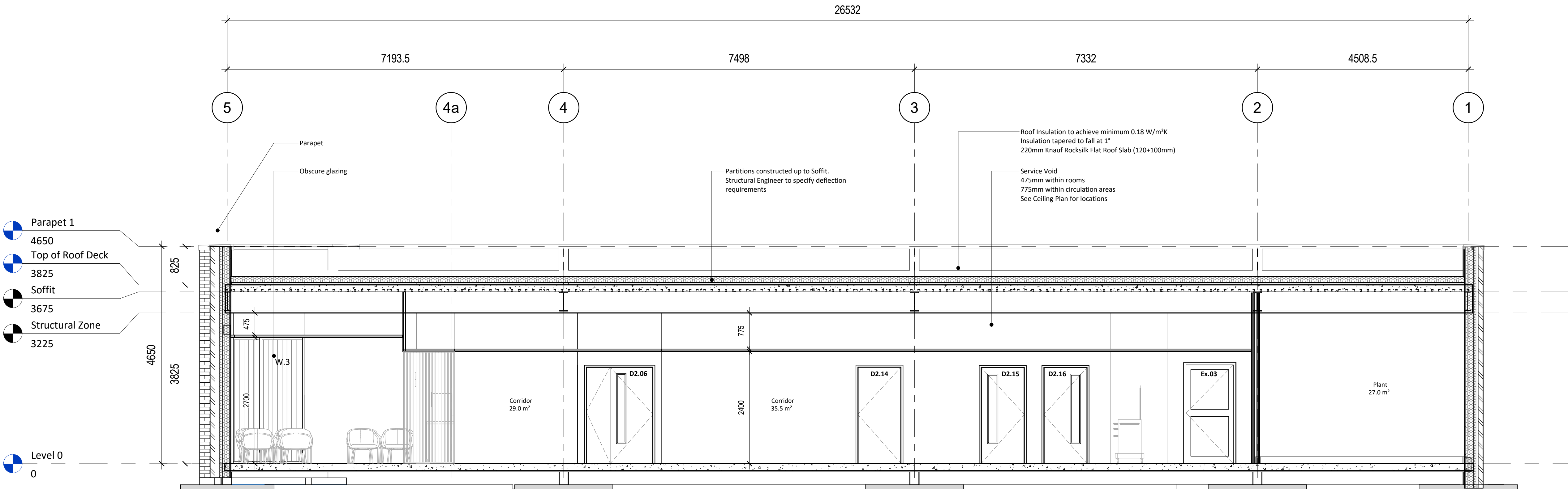
Section D-D 1 : 50
