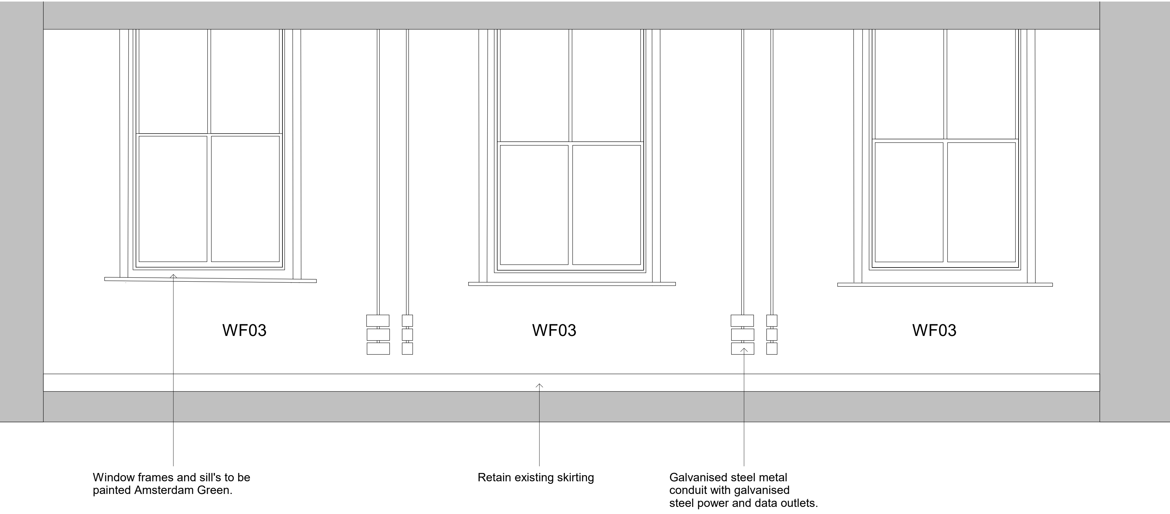
2FL - Elevation 8
