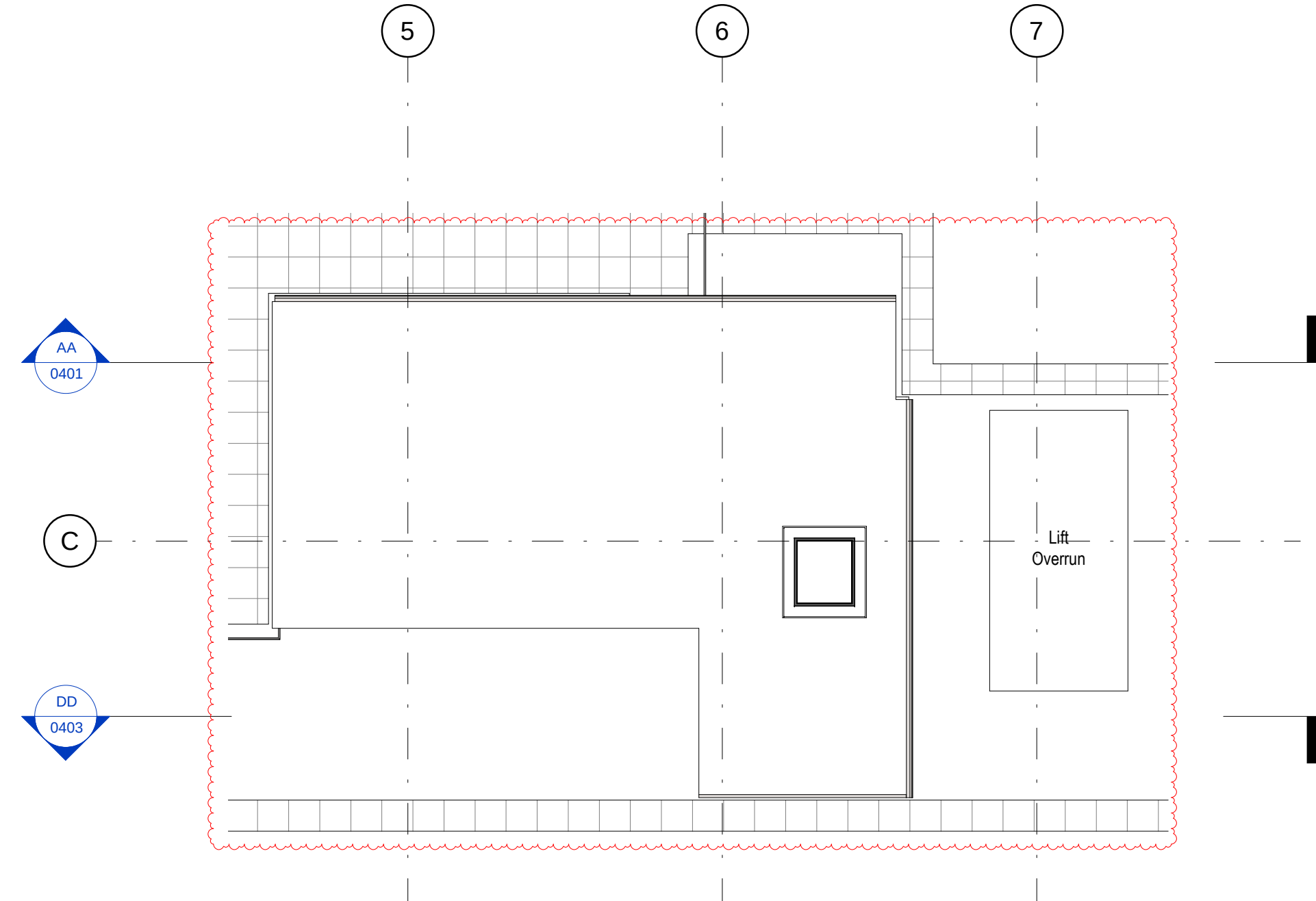
Roof - Level 14 1 : 100
