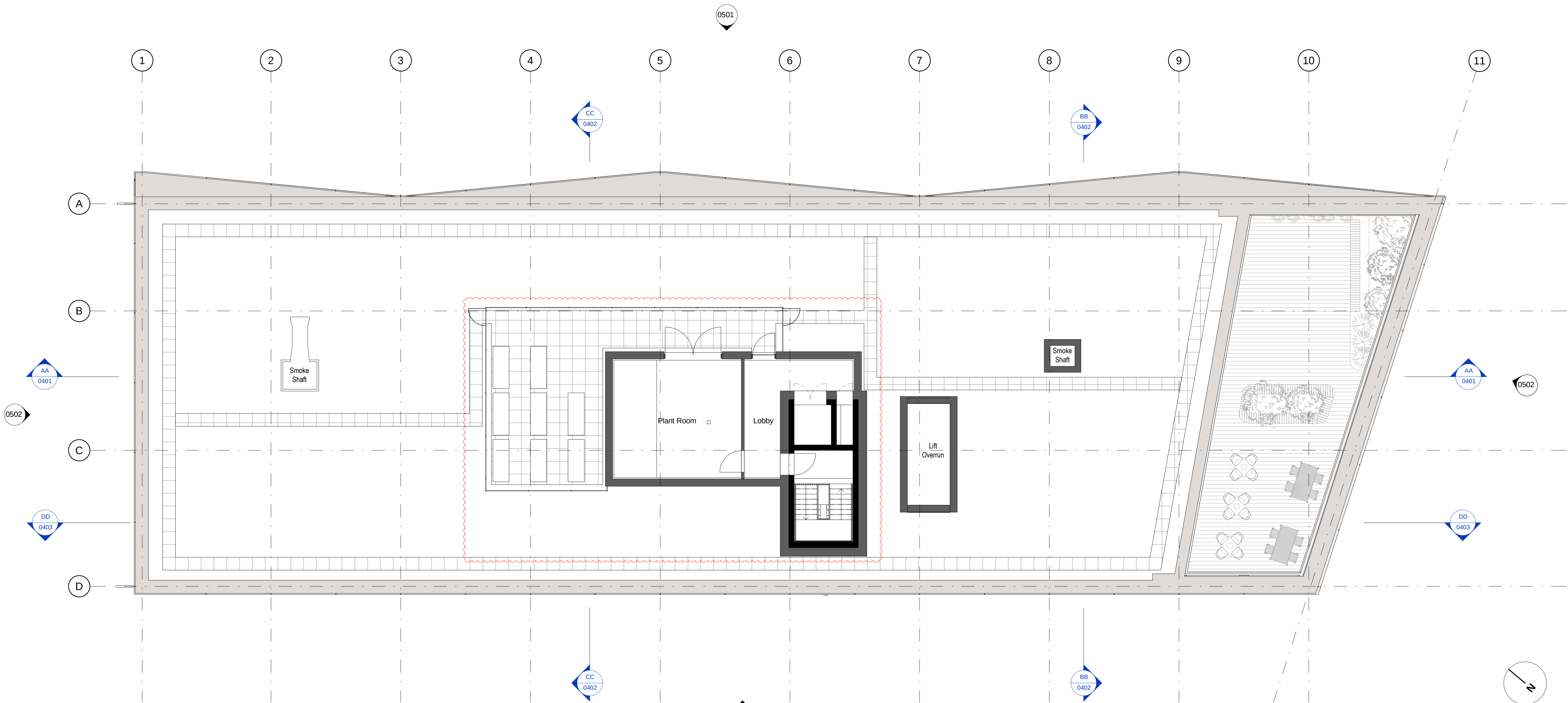
Roof - Level 13 1 : 100
