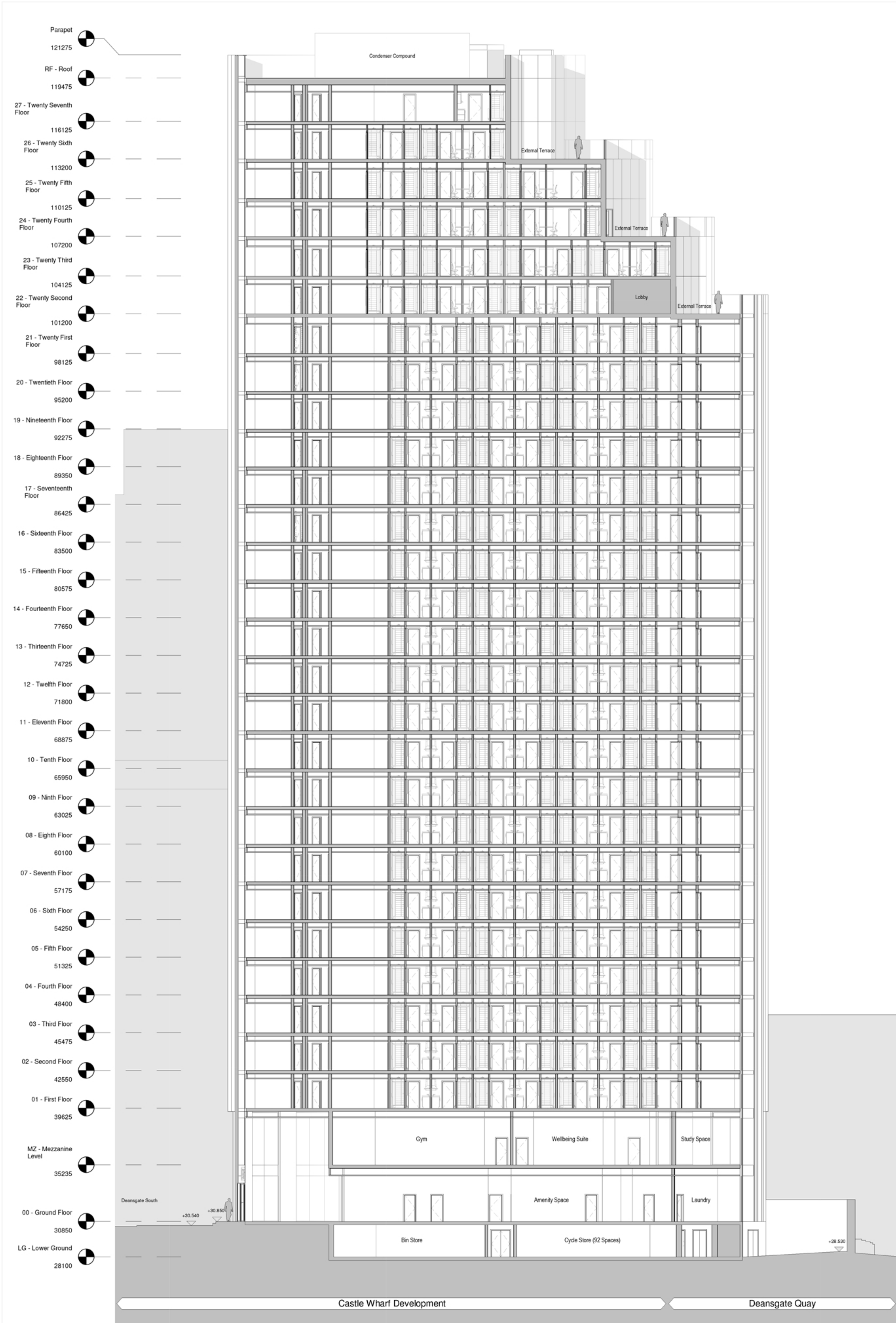
01 Section A-A 1 : 200
