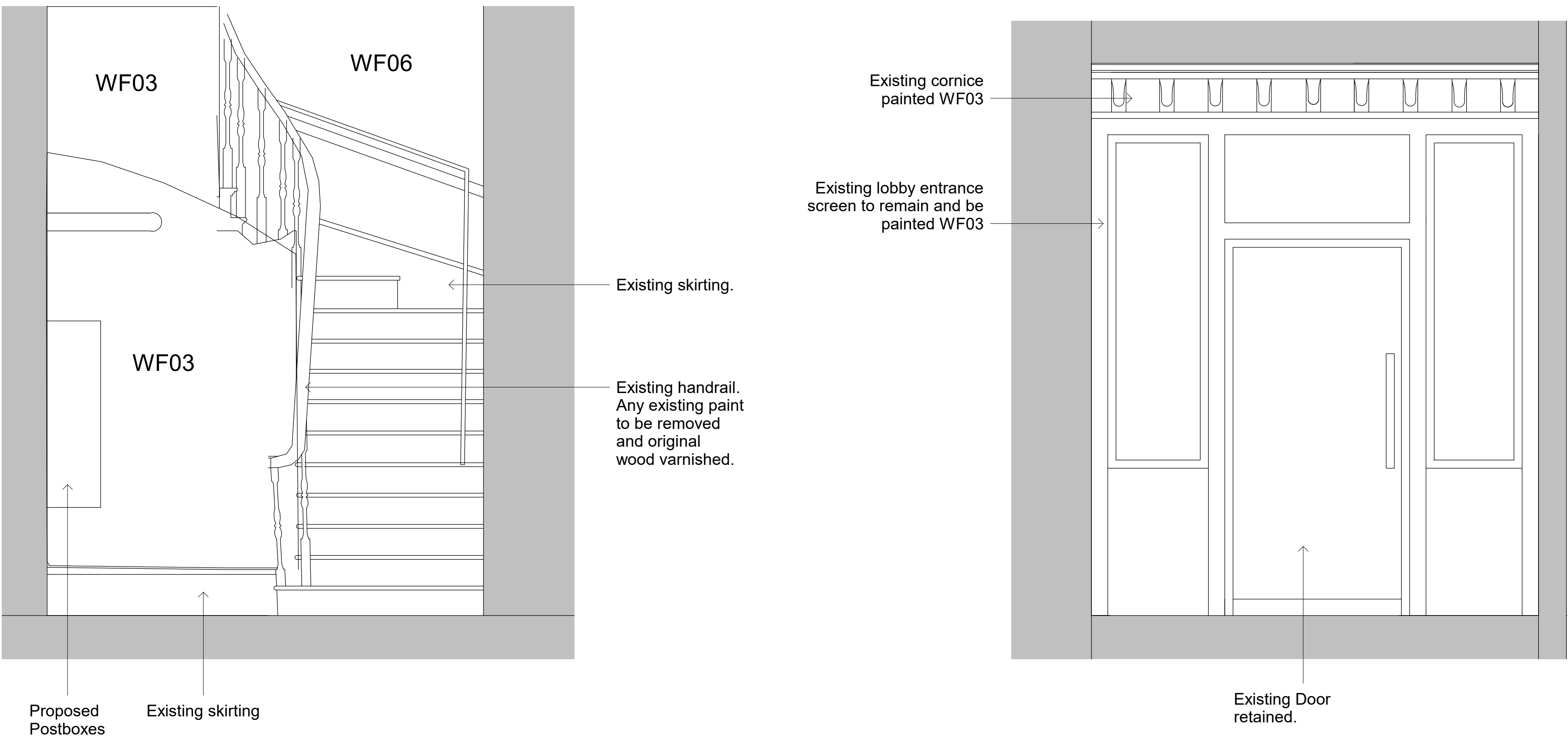
GFL - Elevation 2 1 : 20
