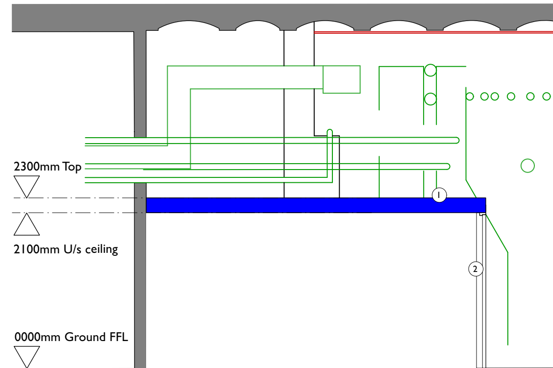
4 Section BB Scale: 1:50
