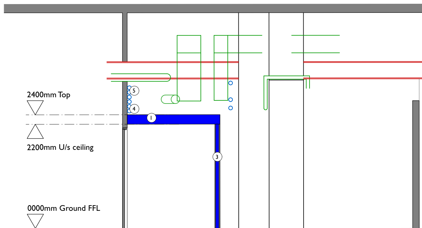
3 Section AA Scale: 1:50
