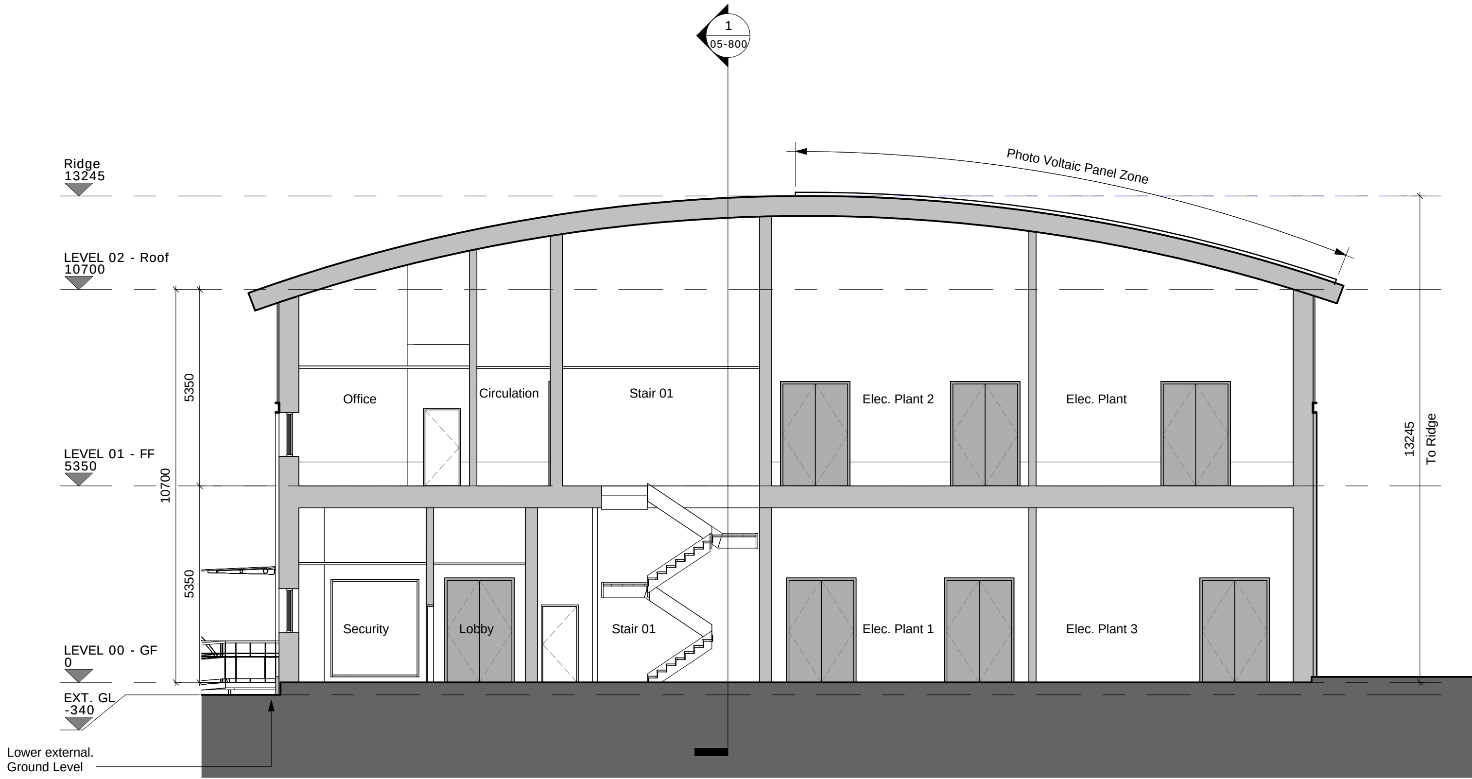
2 05-Section 2 1 : 100
