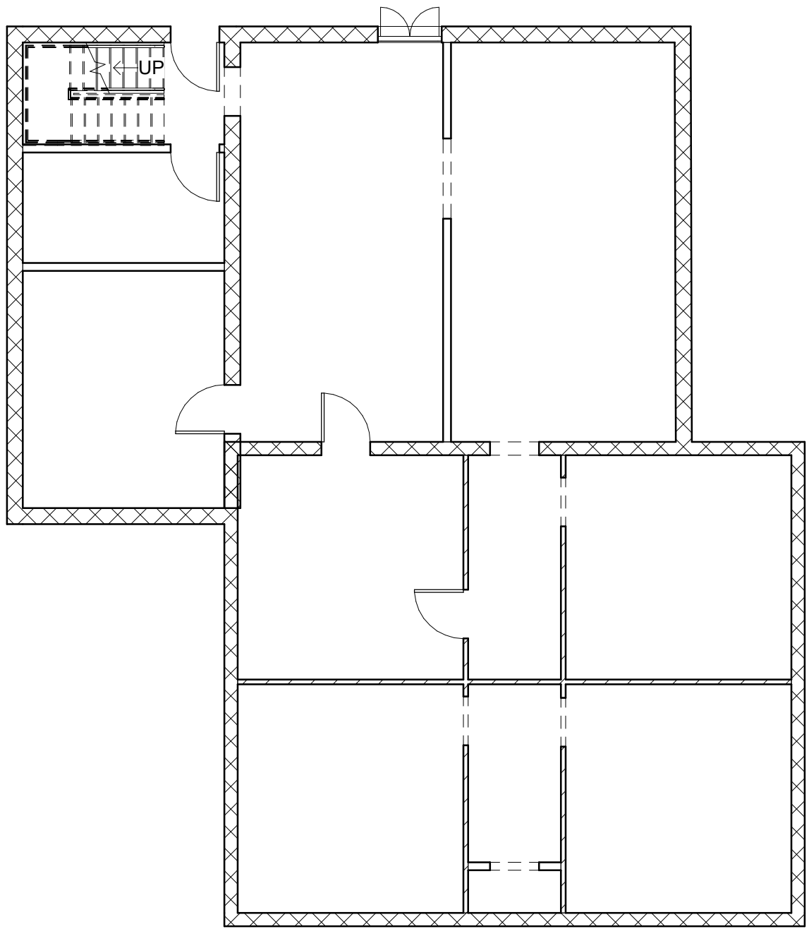
1 Basement - Existing 1 : 100
