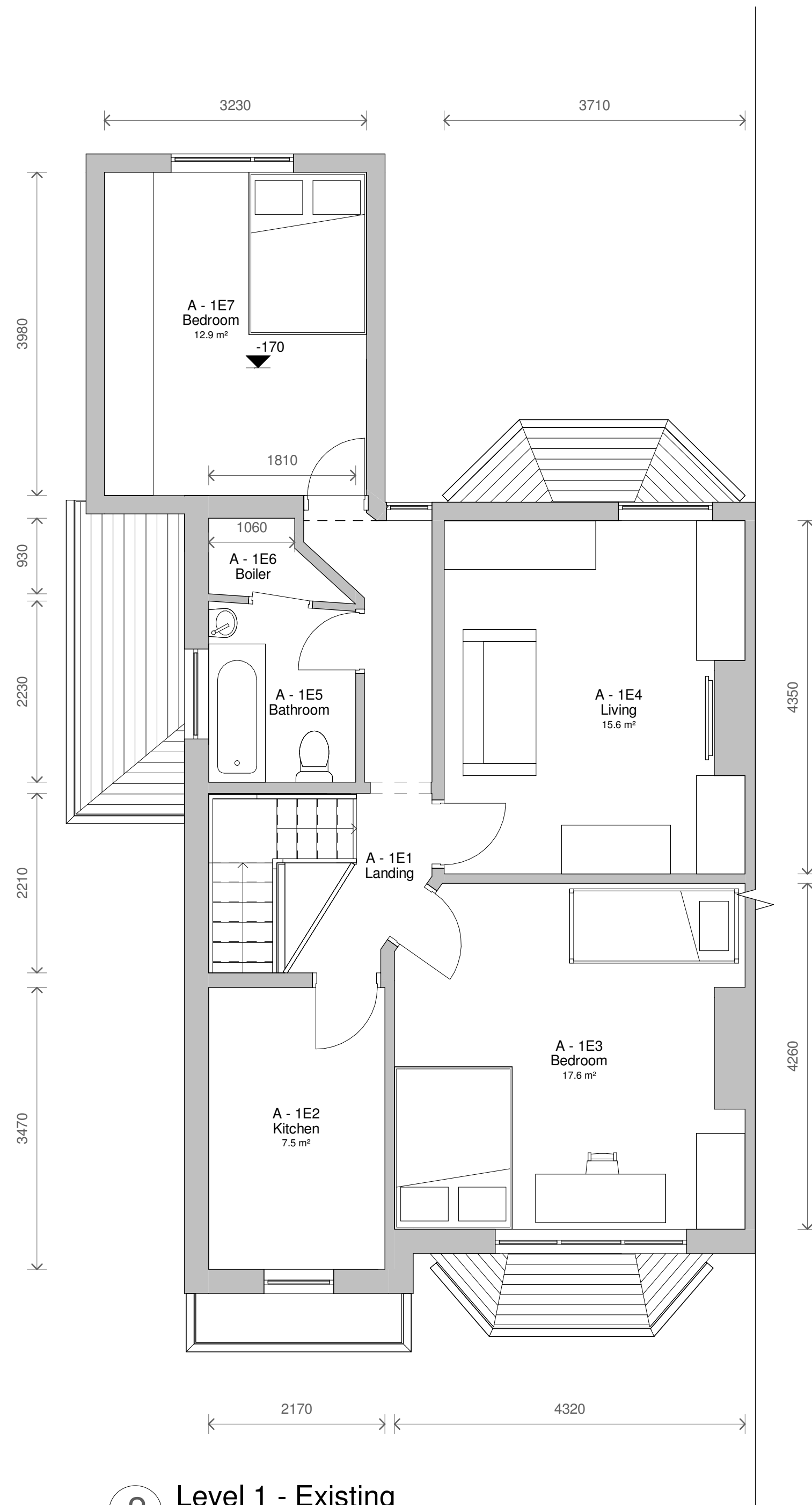
2 Level 1 - Existing 1 : 50
