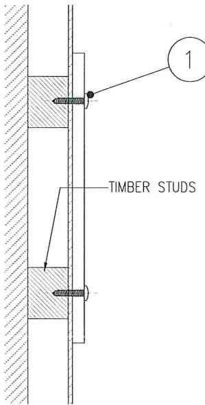
C06c – STUD WALL 32MM SCREWS
