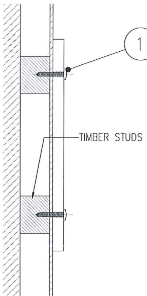
C06d – STUD WALL 38MM SCREWS
