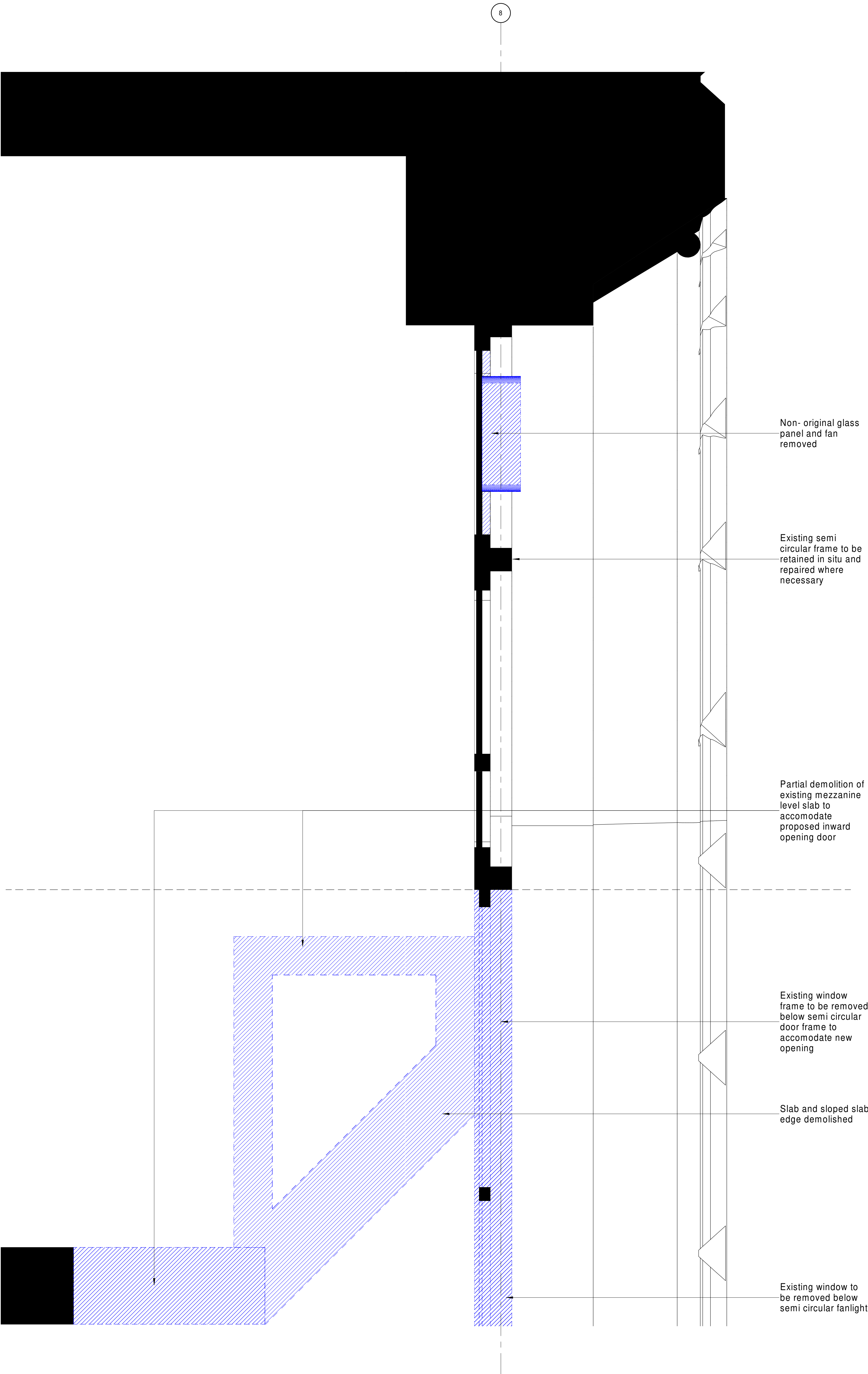
3 External Door Type D - Demolition Section 32651 1:5
