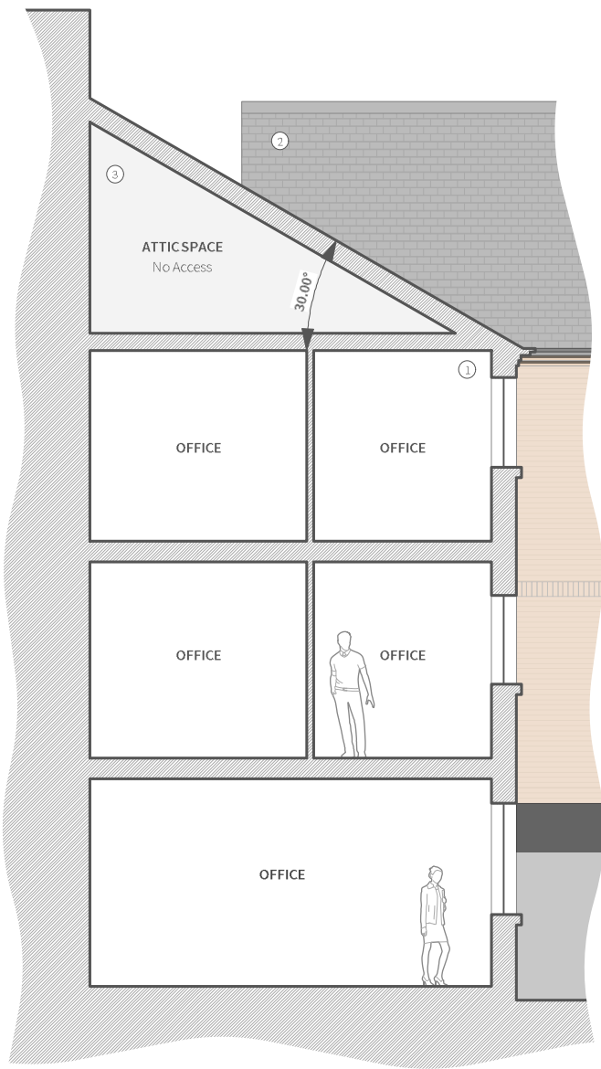
SECTION A-A 1:100
