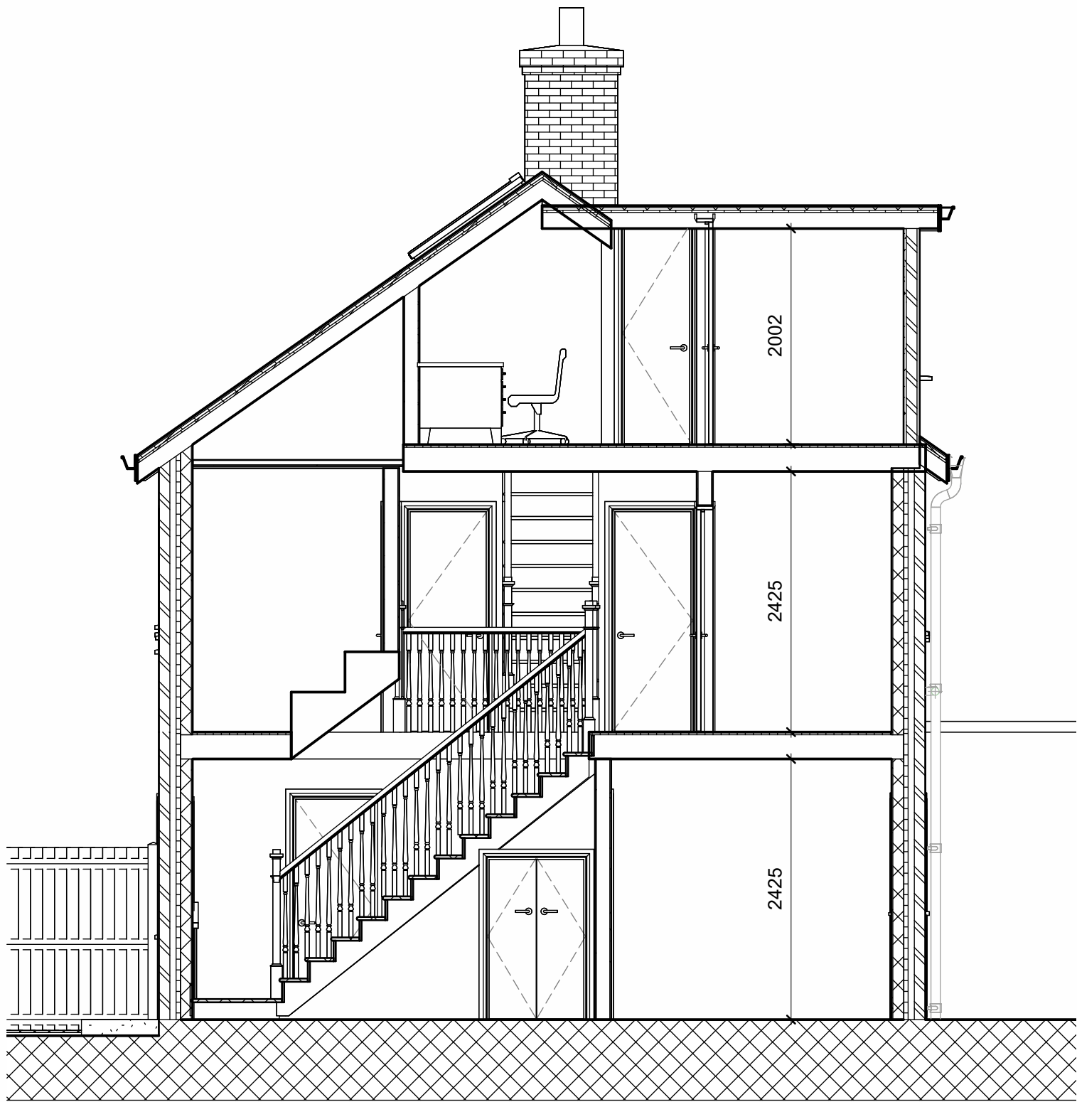
Section A-A' 1 : 50
