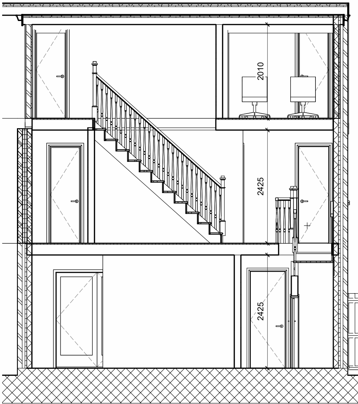
Section B-B' 1 : 50
