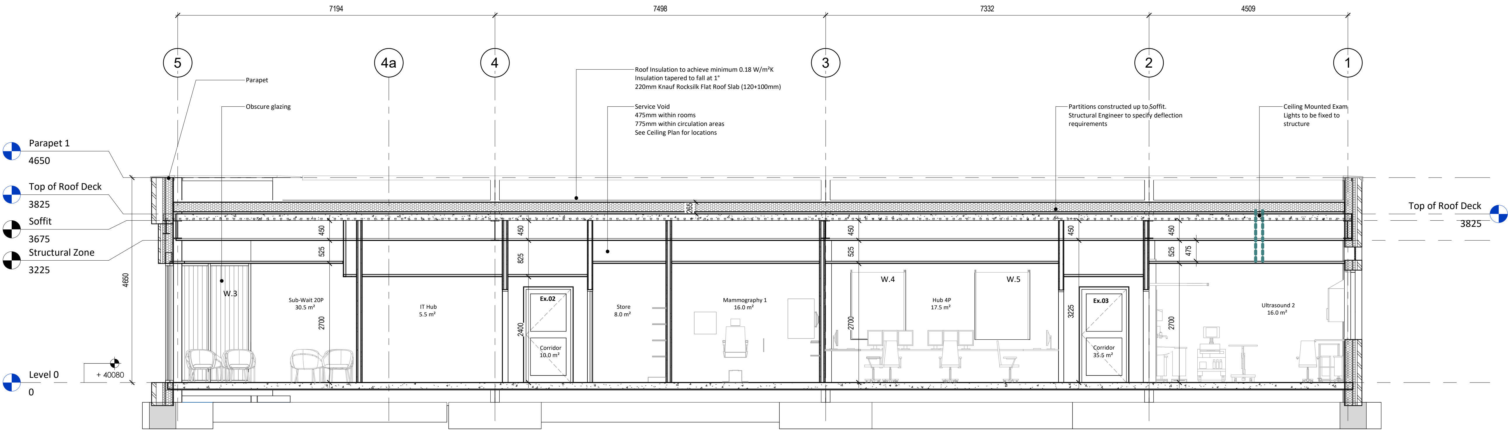
Section B-B 1 : 50
