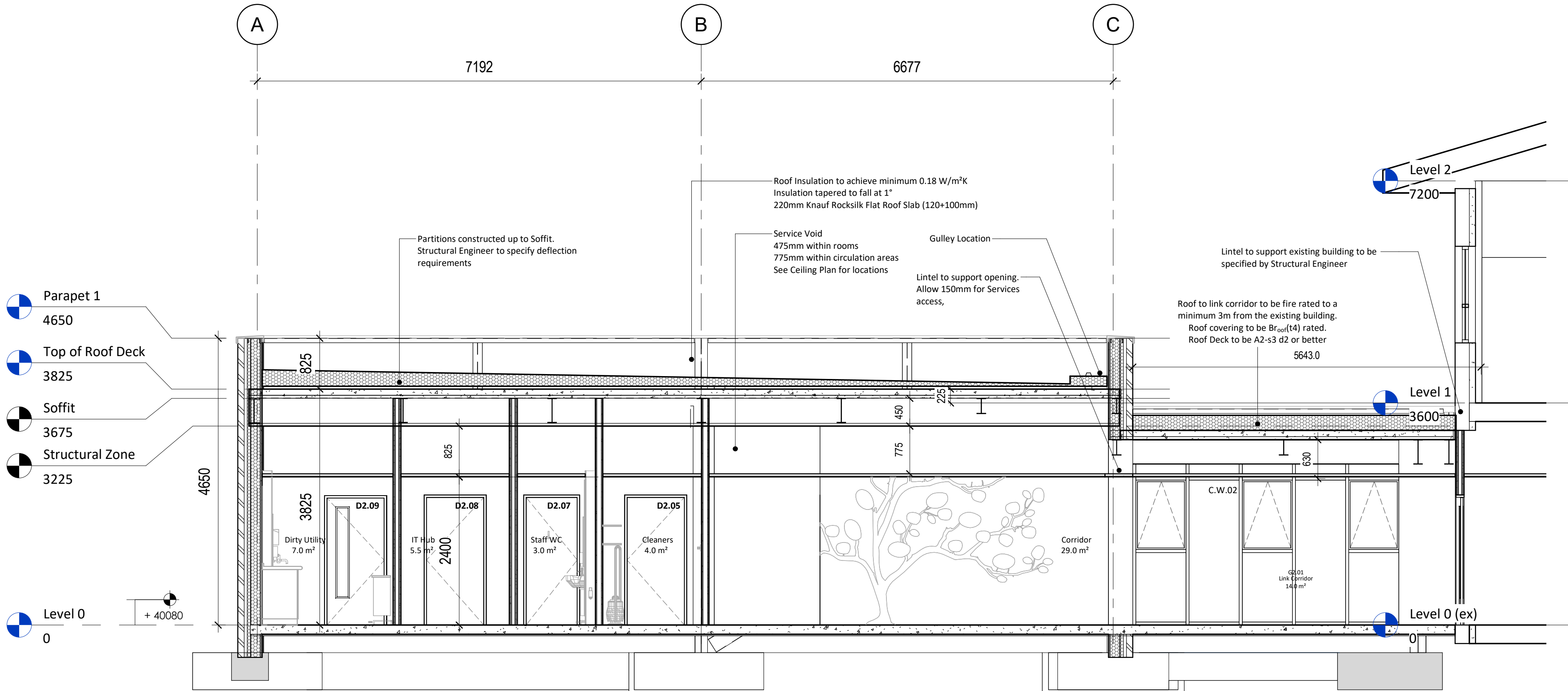
Section A-A 1 : 50
