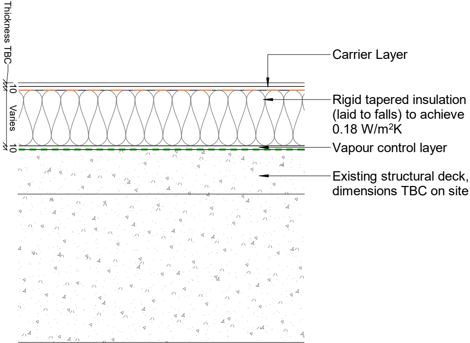
Roof Type 1 1 : 10
