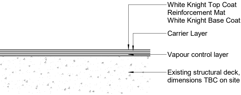
Roof Type 5 1 : 10
