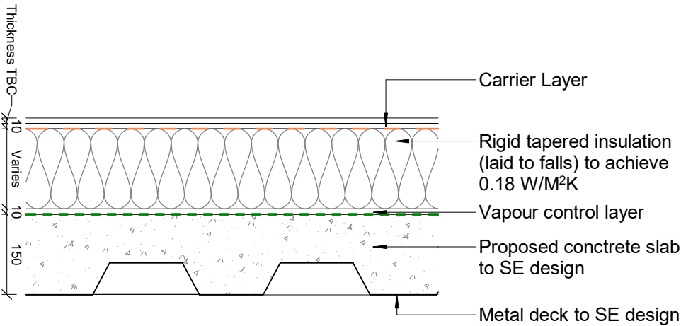
Roof Type 3 1 : 10
