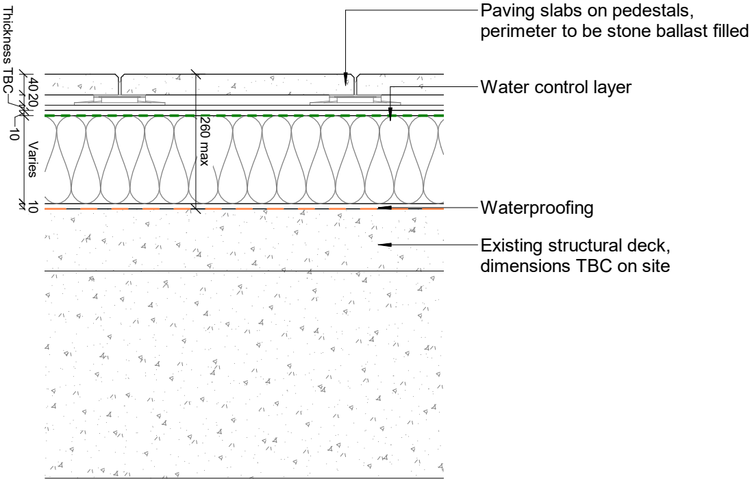
Roof Type 2 1 : 10
