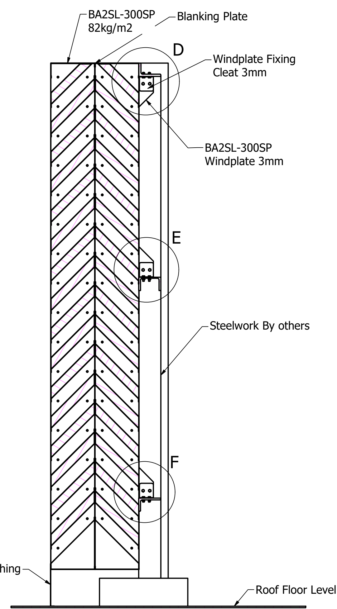
C-C ( 1 : 16 )
