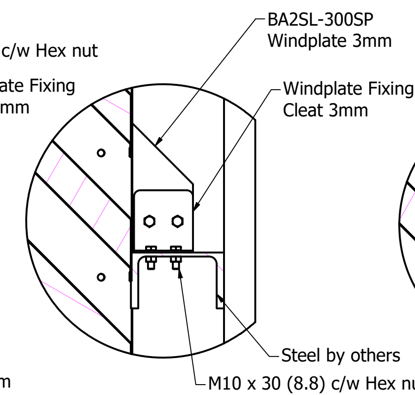
E ( 1 : 6 )
