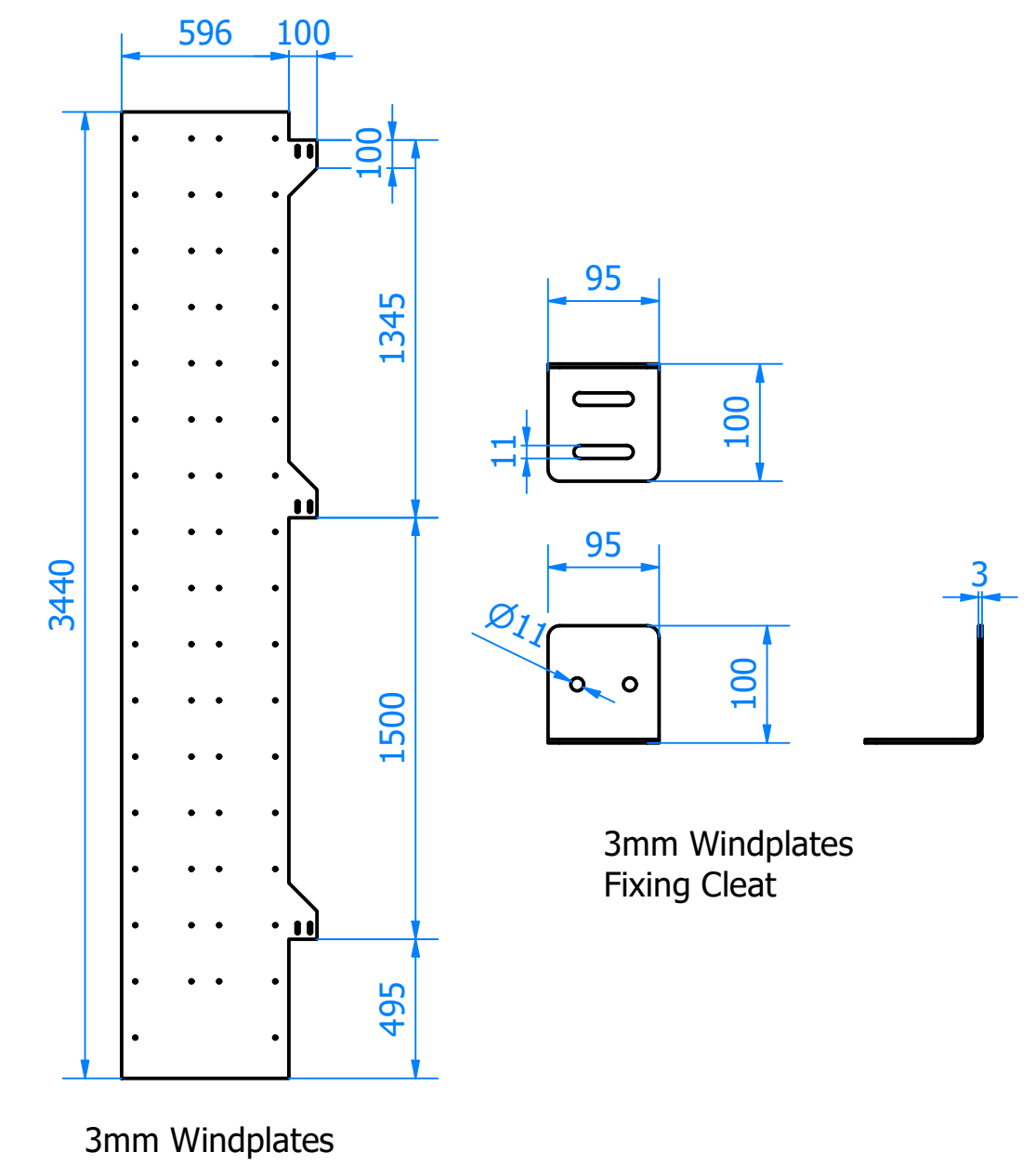
F ( 1 : 6 )
