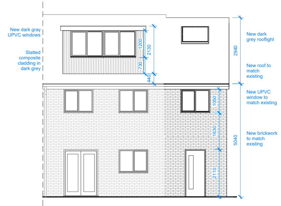
3 Rear 1 : 100
