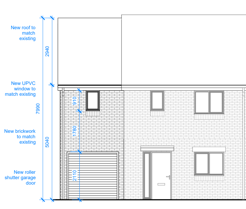
1 Front 1 : 100
