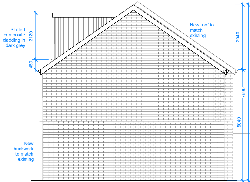
2 Side 1 : 100
