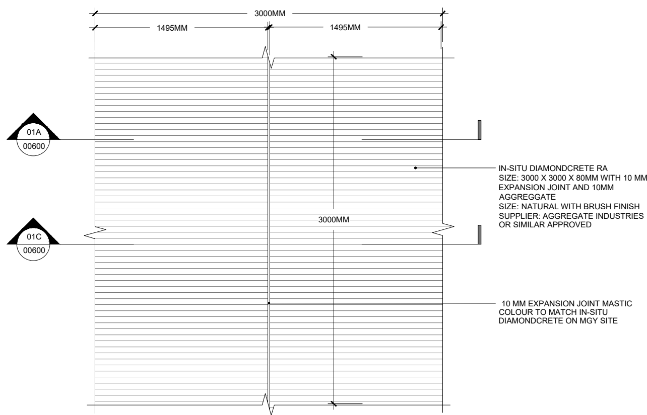
01B 00600 ST01: IN-SITU DIAMONDCRETE RA PLAN
