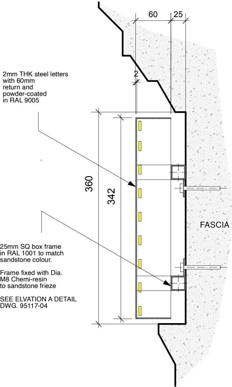
SECTION A-A - 1:4
