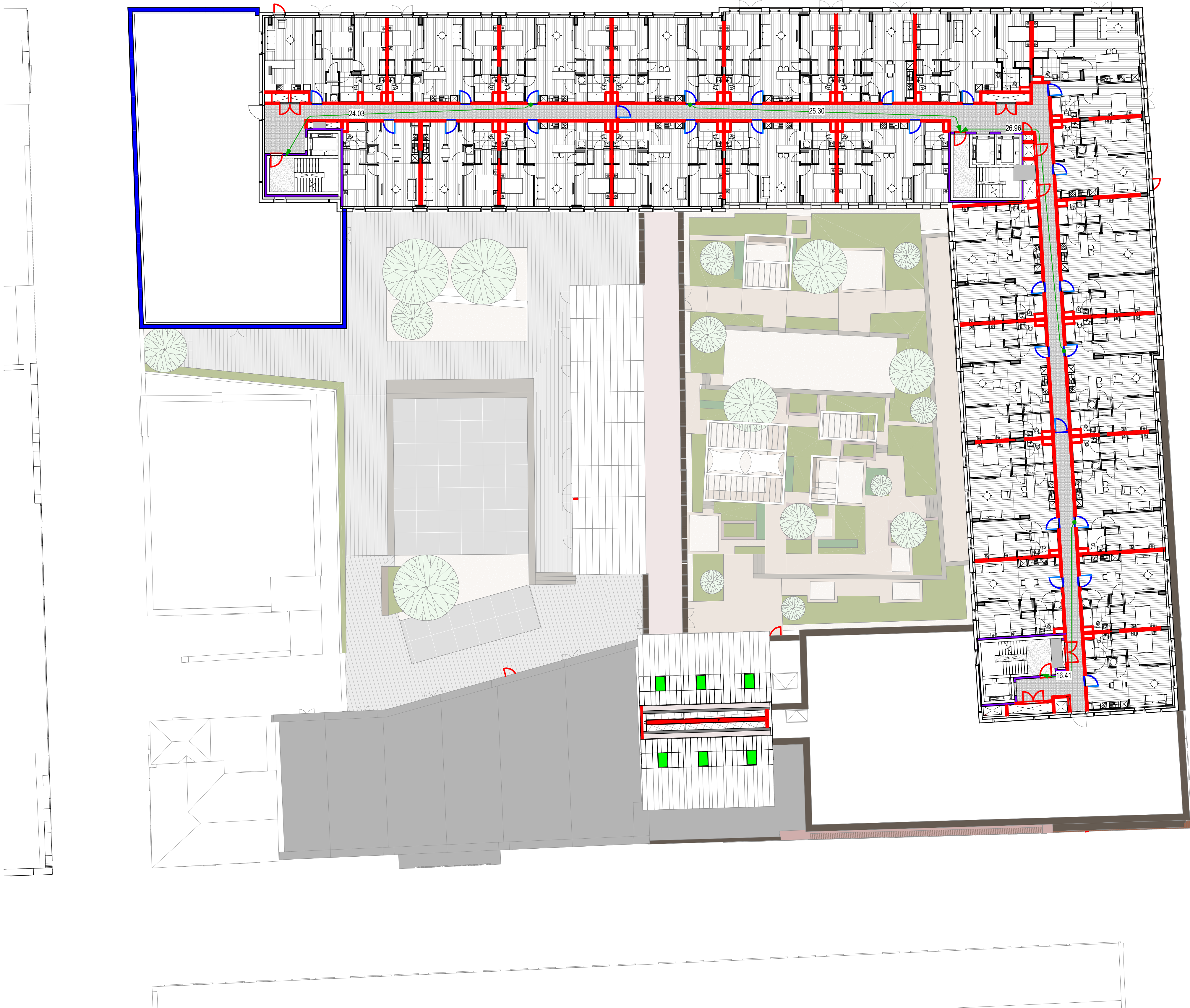
FIRE PLAN LEVEL 06 SCALE: 1 : 200
