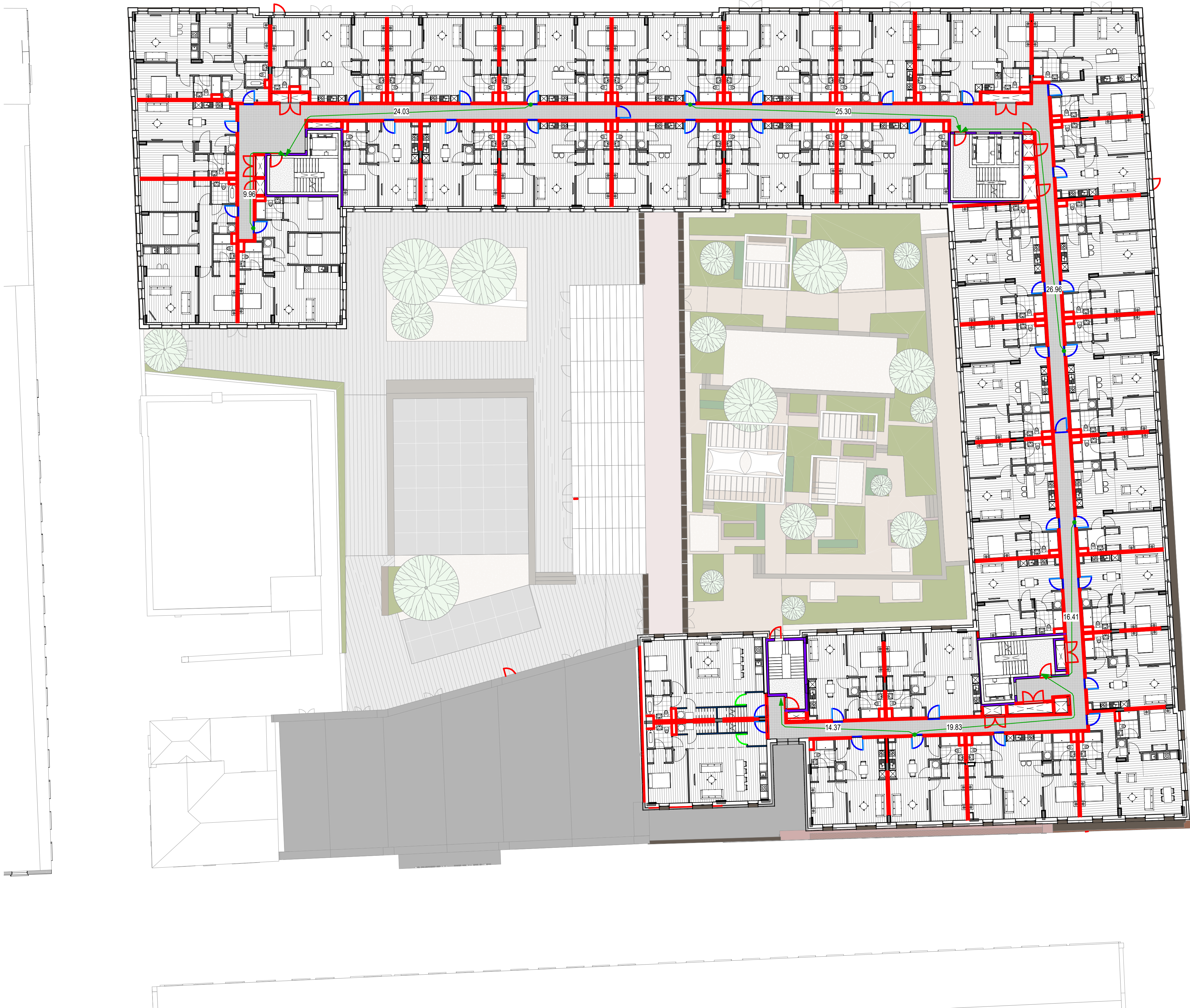
FIRE PLAN LEVEL 04 SCALE: 1 : 200
