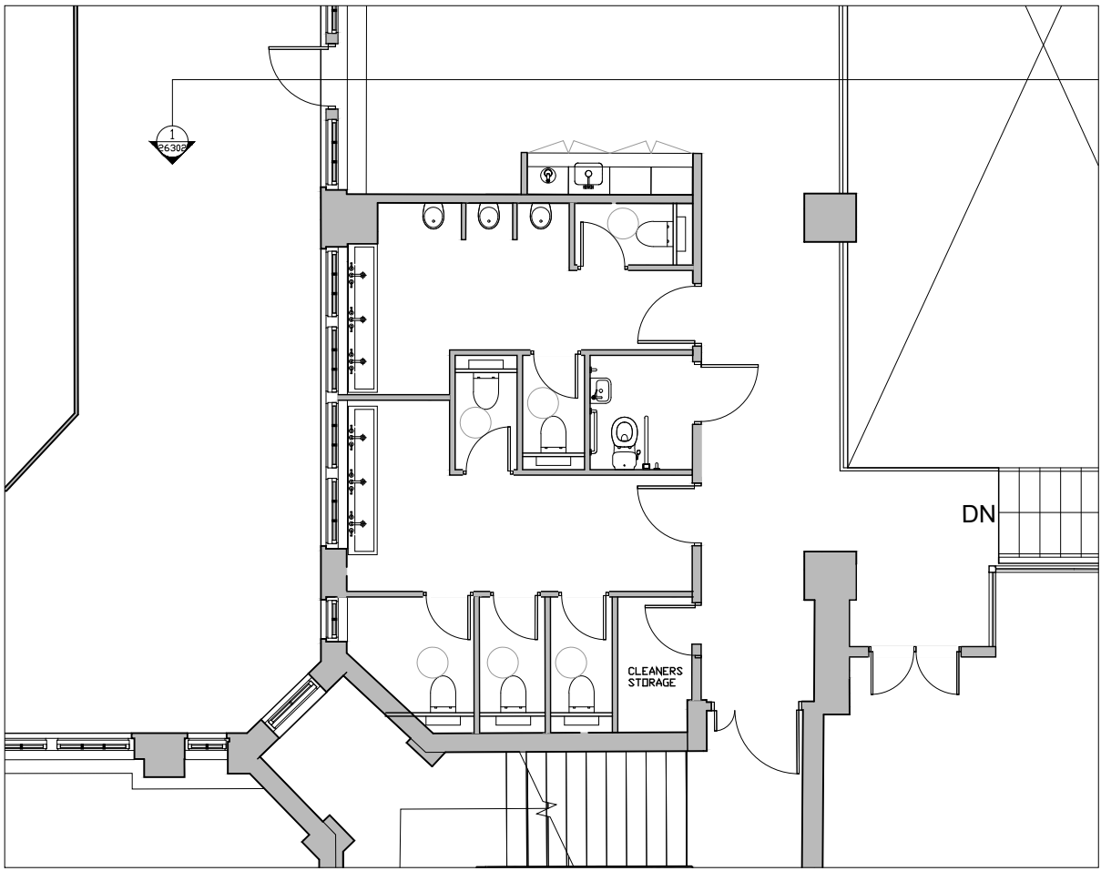
Level 01 WC - 1:100
