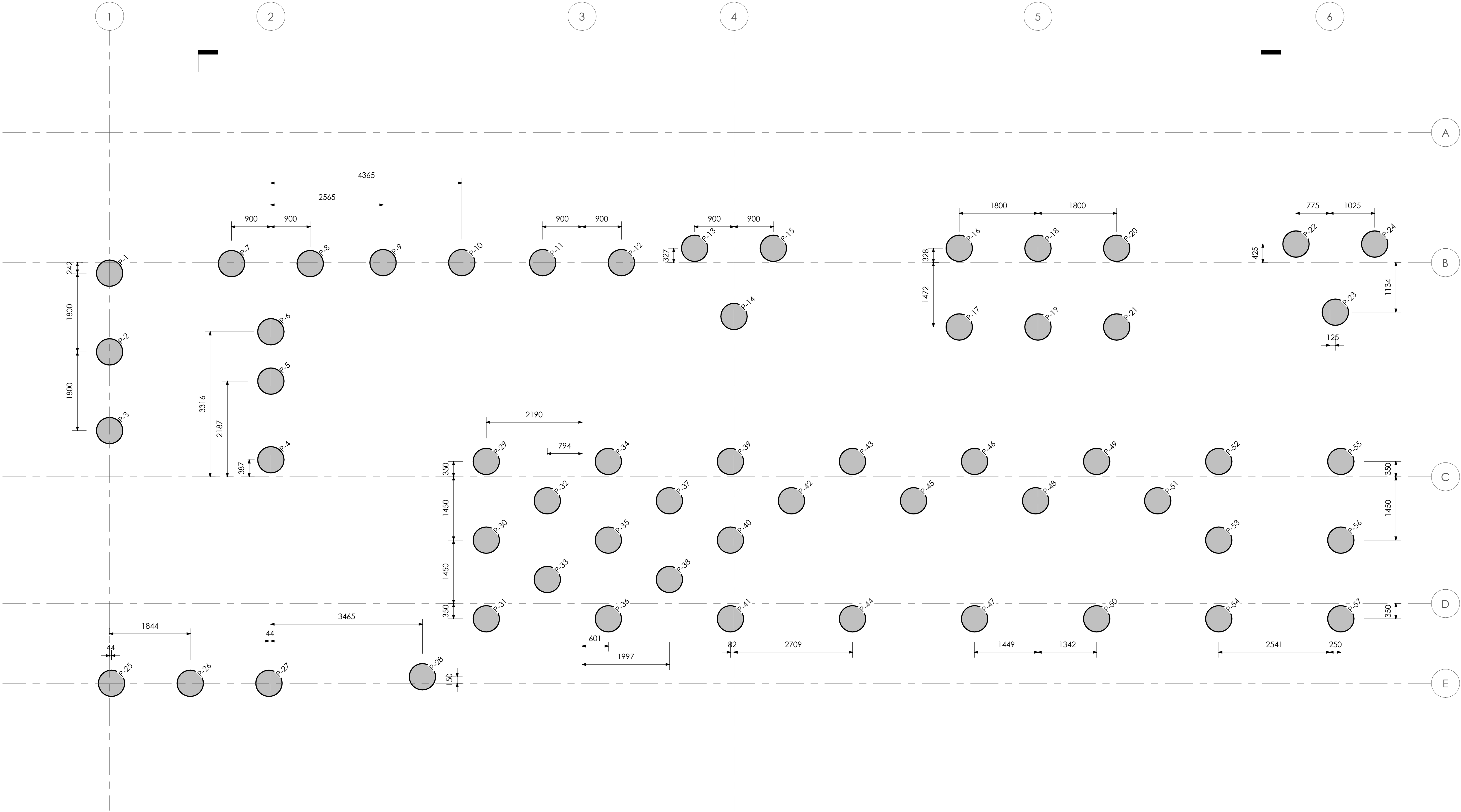
PILING LAYOUT 1 : 50
