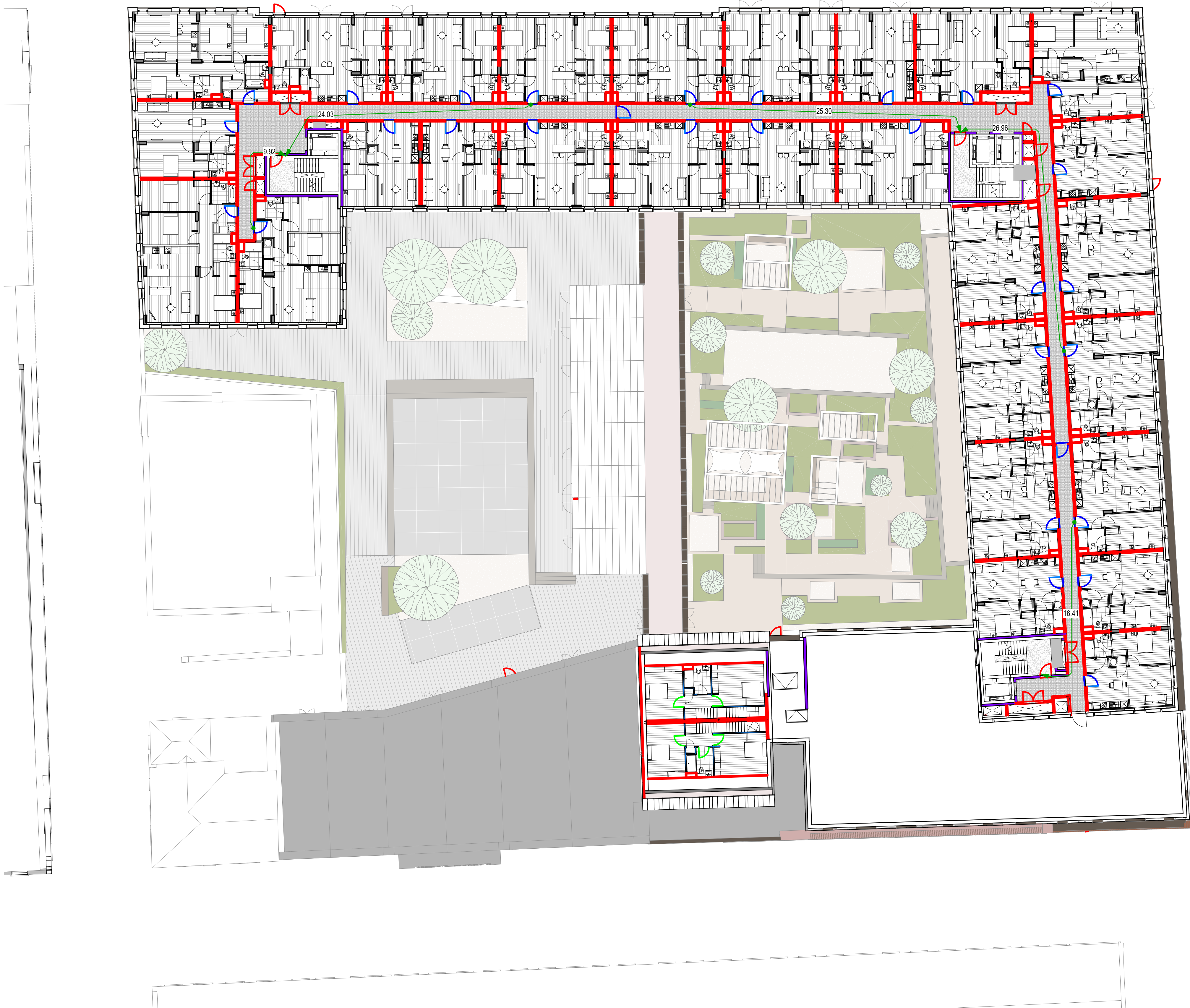
FIRE PLAN LEVEL 05 SCALE: 1 : 200
