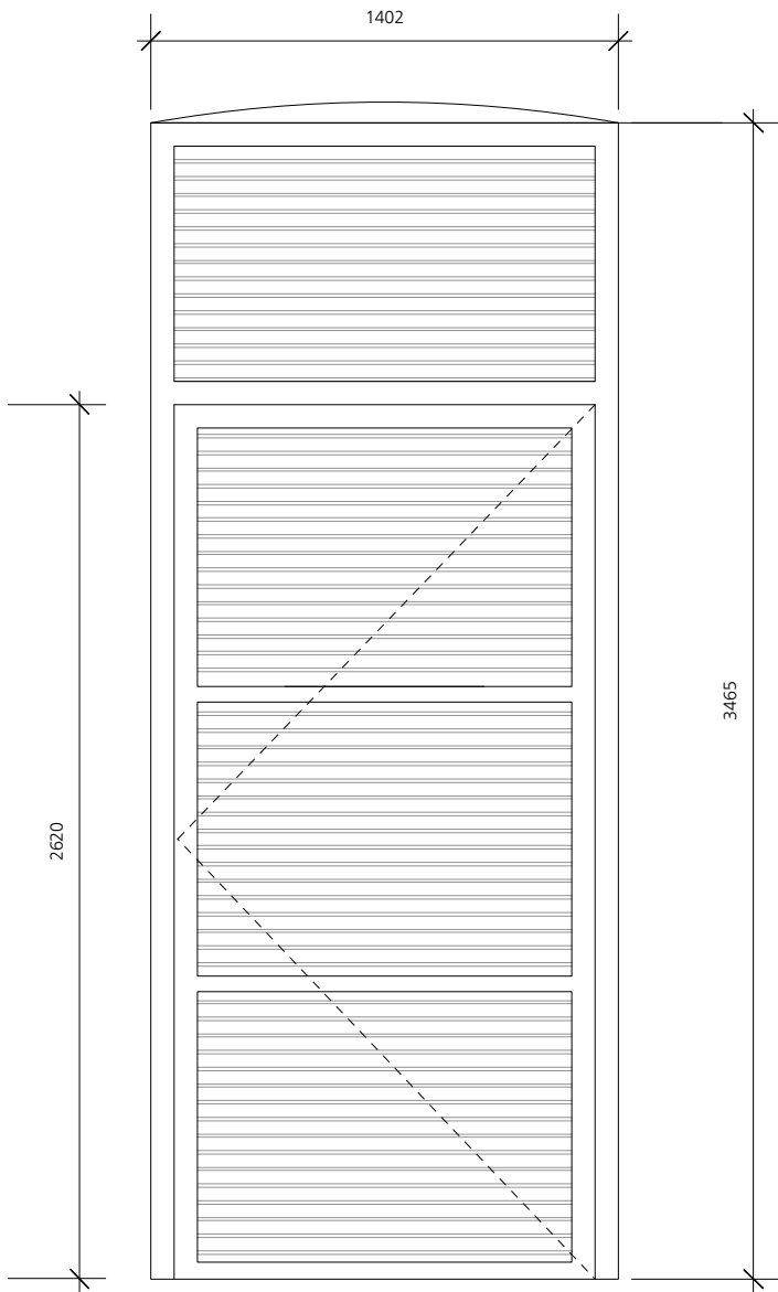
DOOR TYPE AD4
