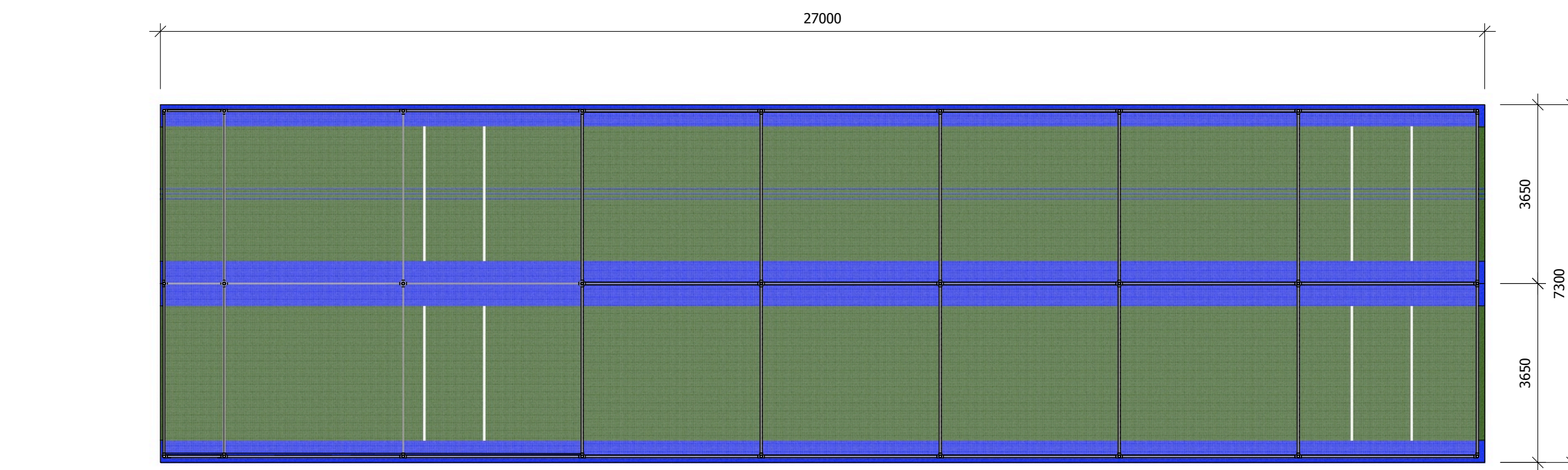
PLAN scale: 1:100
