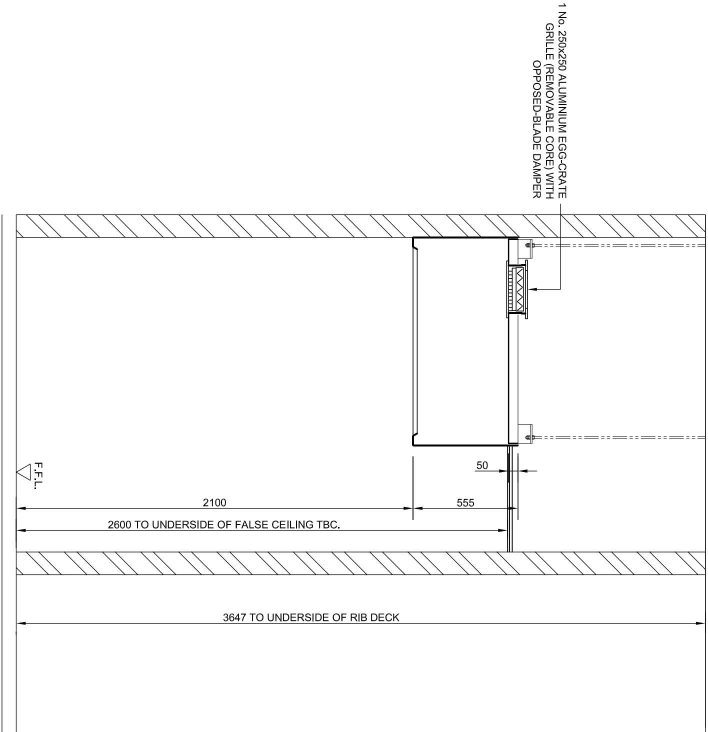
SECTION A-A
