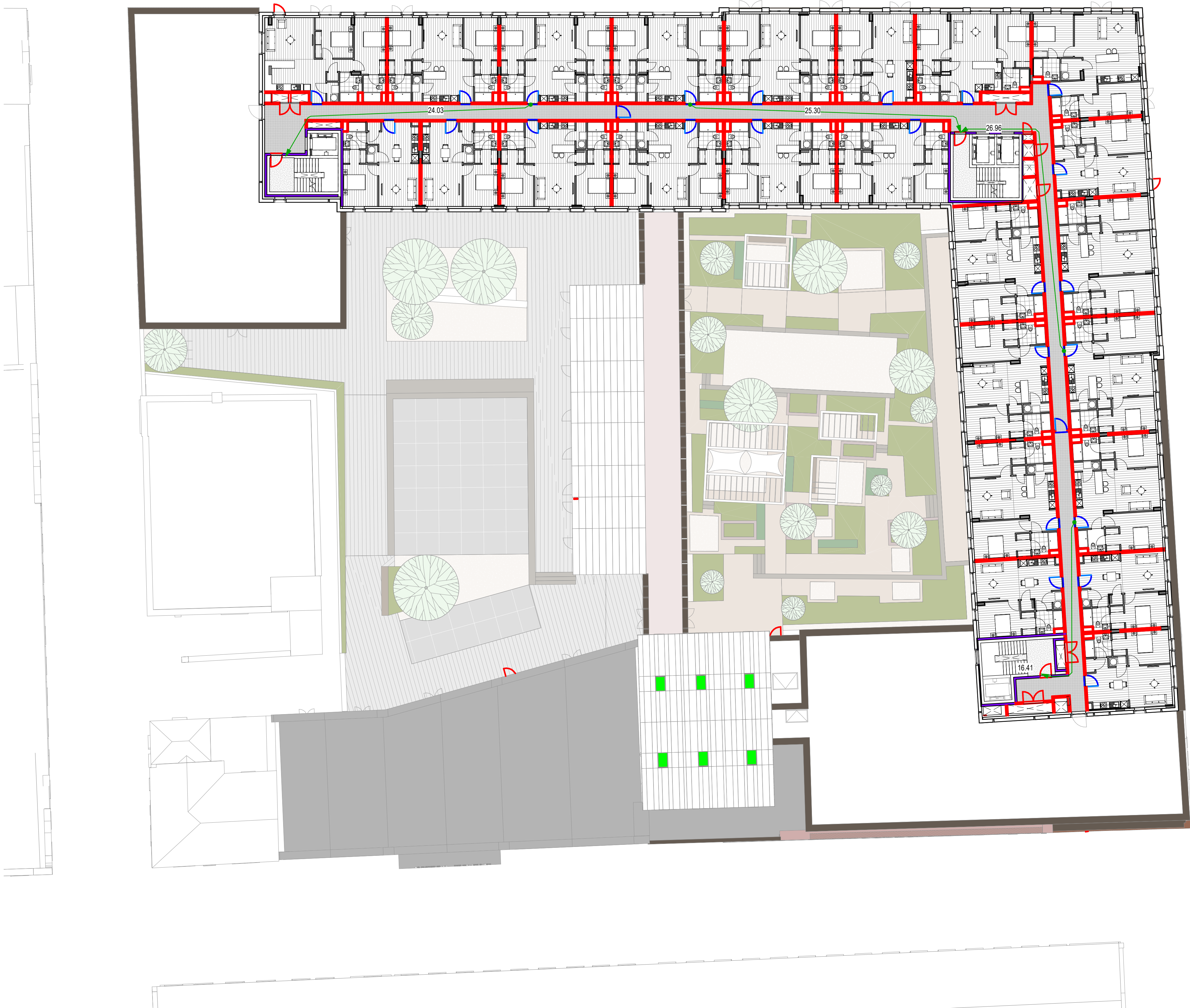
FIRE PLAN LEVEL 07 SCALE: 1 : 200
