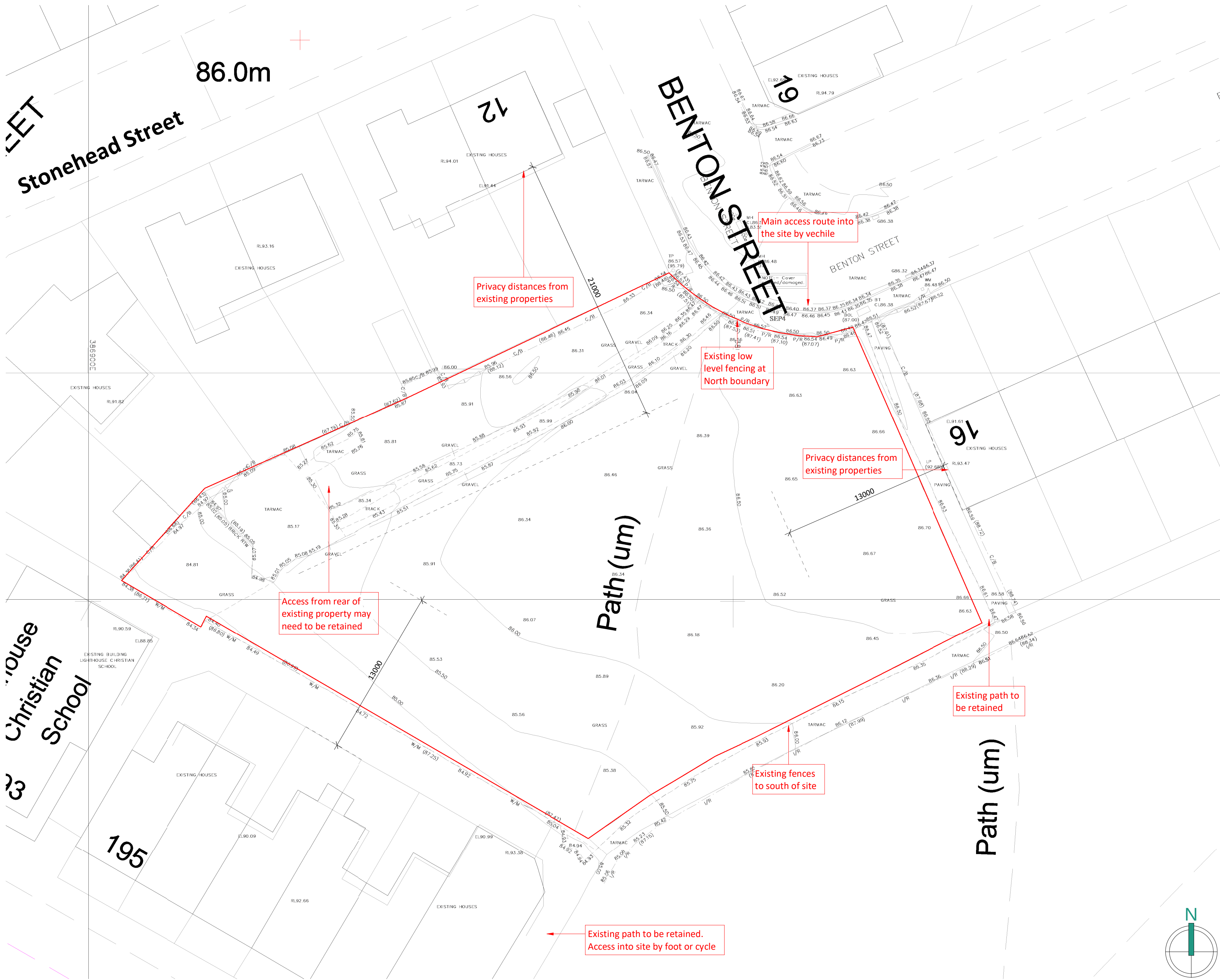
01 - Constraints Plan 1 : 200
