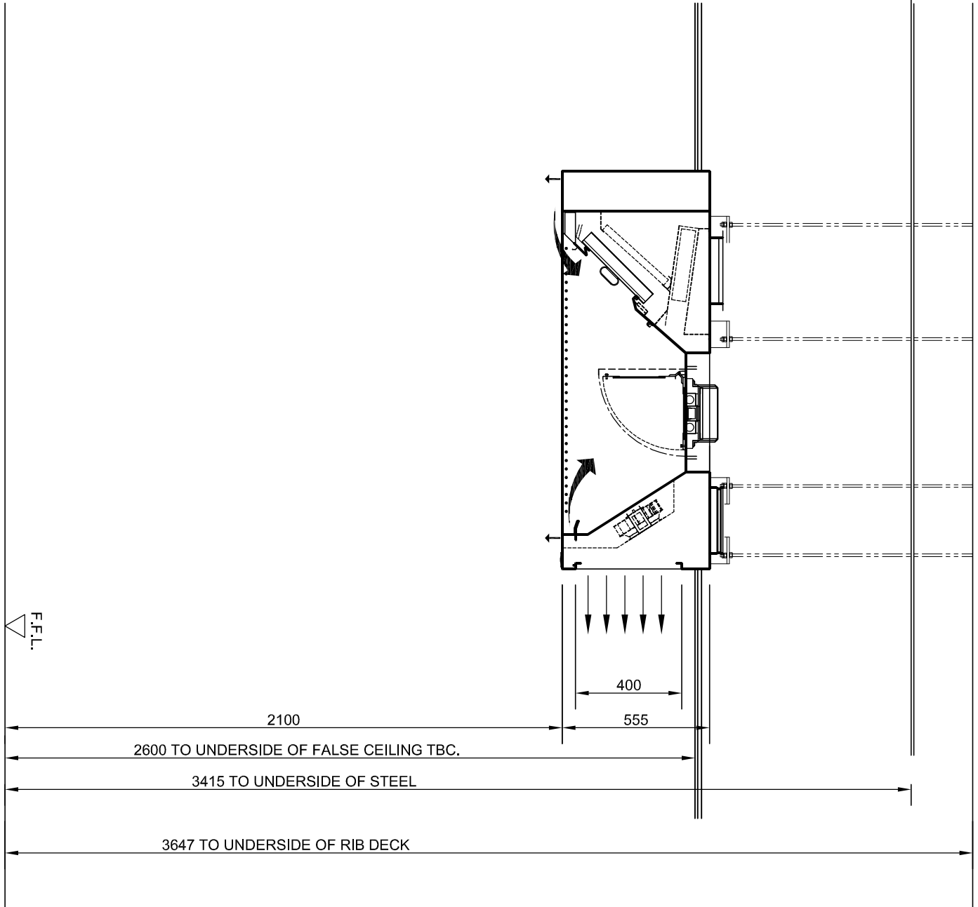
SECTION A-A
