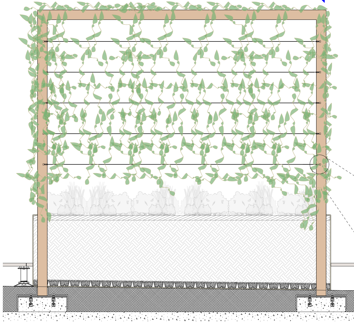
2 Pergola Detail Section B-B' Scale: 1:20
