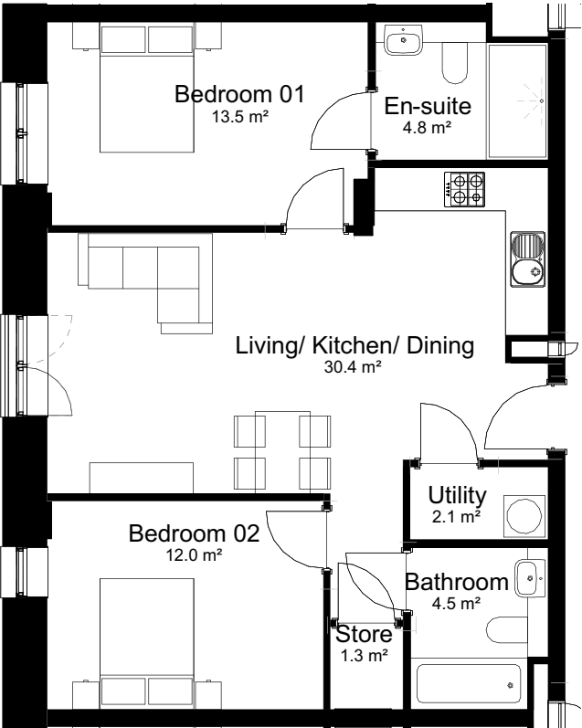
Type B2 / B3 / B4 / B7 1:100
