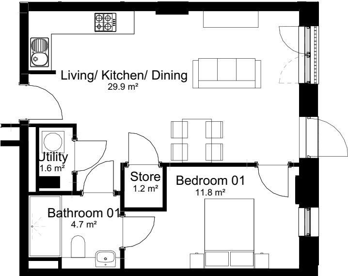
Type A5 1 : 100
