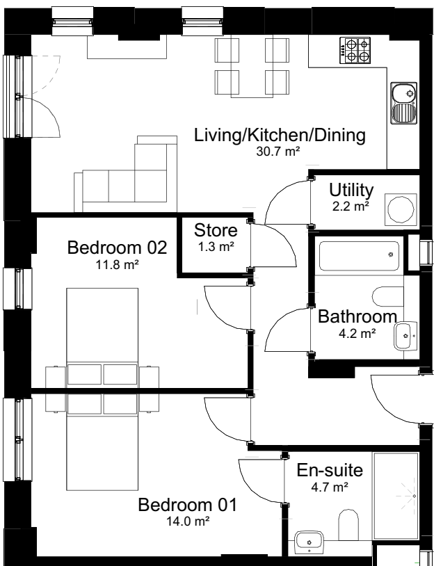
Type B10 1 : 100
