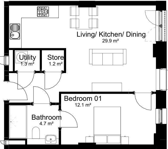
Type A4 1 : 100
