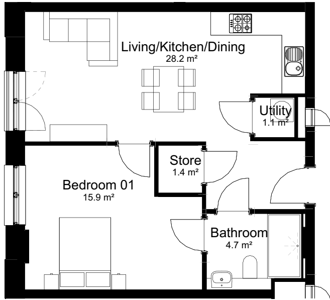
Type A1 / A6 1 : 100
