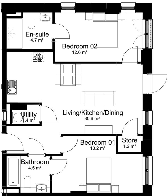
Type B9 1 : 100
