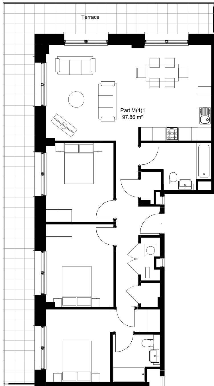
Type 15 - 3b6p 1 : 100
