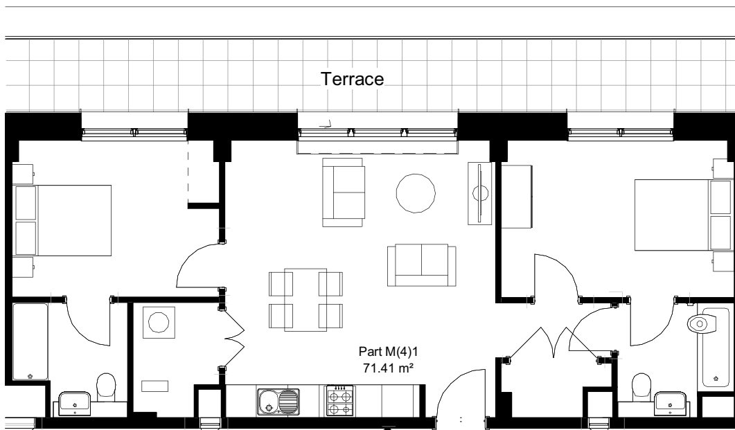
Type 14 - 2b4p 1 : 100
