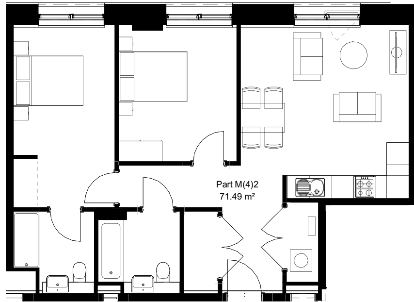
Type 10 - 2b4p 1 : 100
