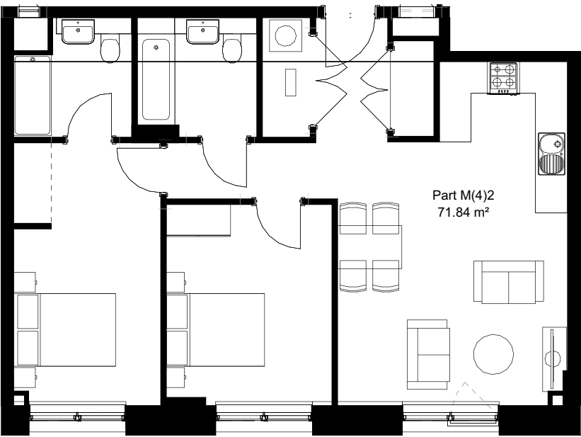
Type 9 - 2b4p 1 : 100
