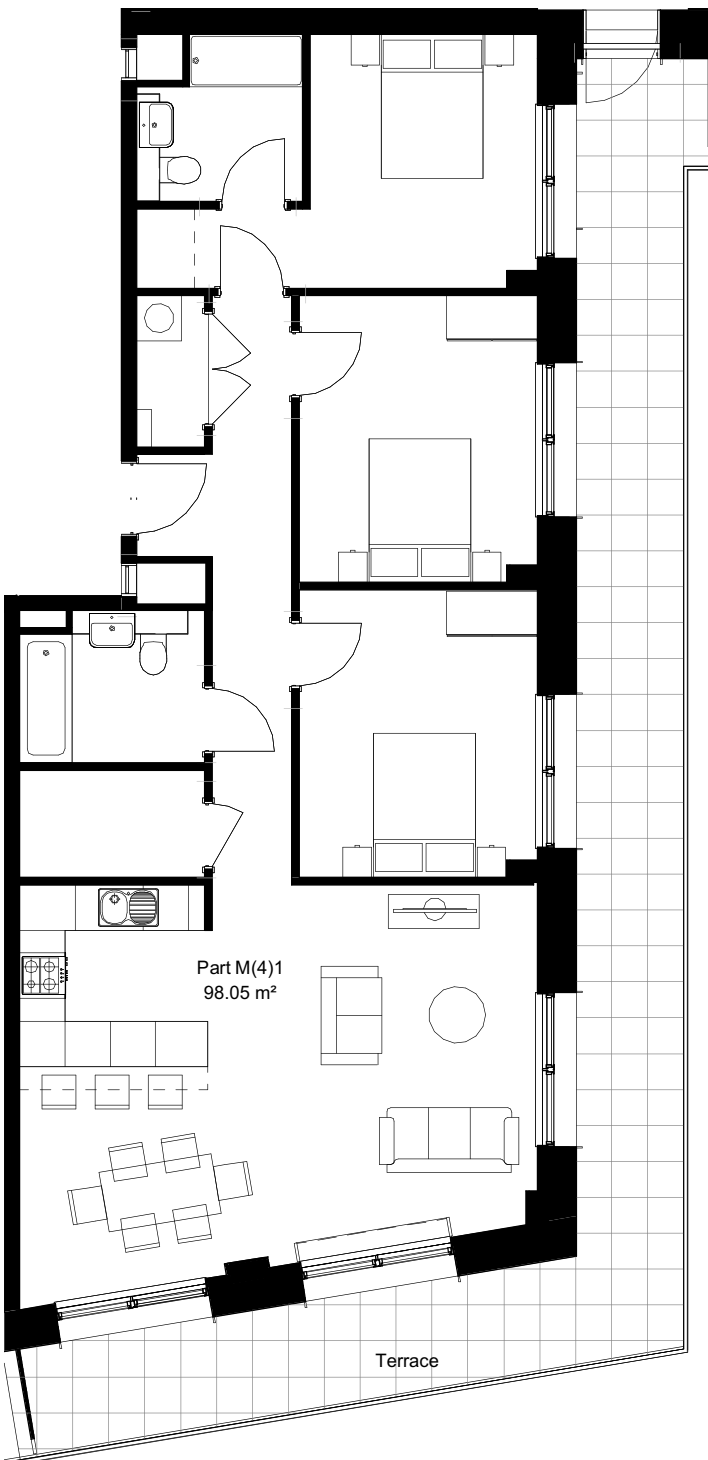
Type 17 - 3b6p 1 : 100
