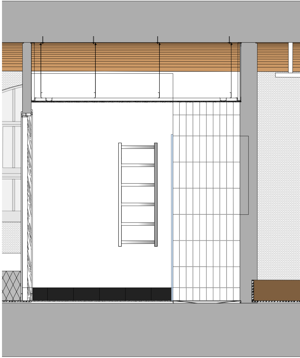
ELEVATION O
