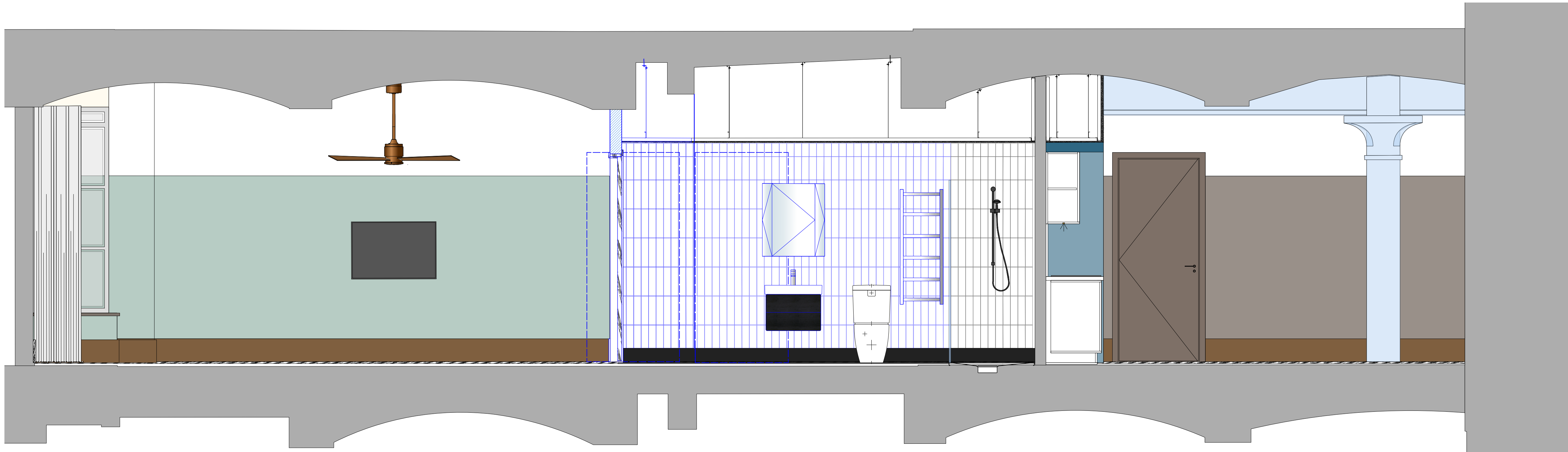
ELEVATION B
