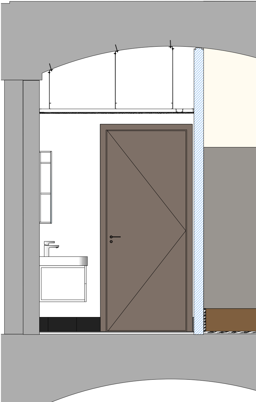
ELEVATION N
