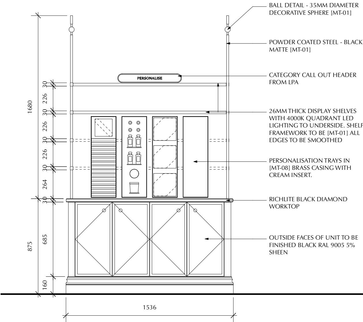
31 Personalisation Wall Display Scale: 1:20
