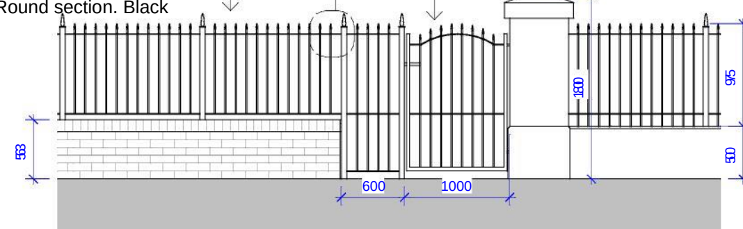
2 Section 1 1 : 50
