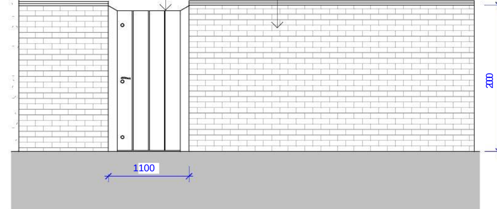
5 Section 3 1 : 50
