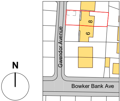
3. Site Block Plan 1 : 1250
