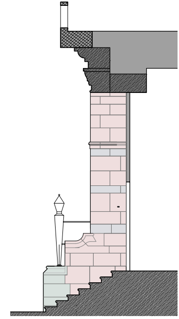
6 Section BB Scale: 1:100
