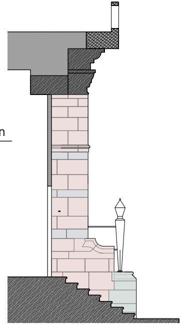
5 Section AA Scale: 1:100
