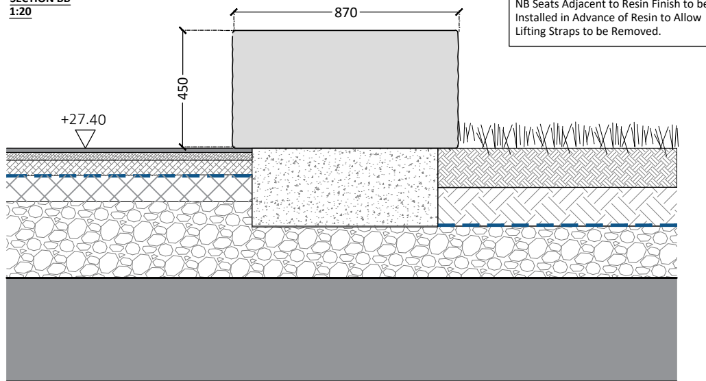
SECTION BB 1:20
