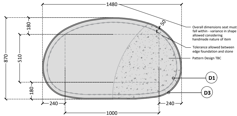
F6 Plan 1:20
