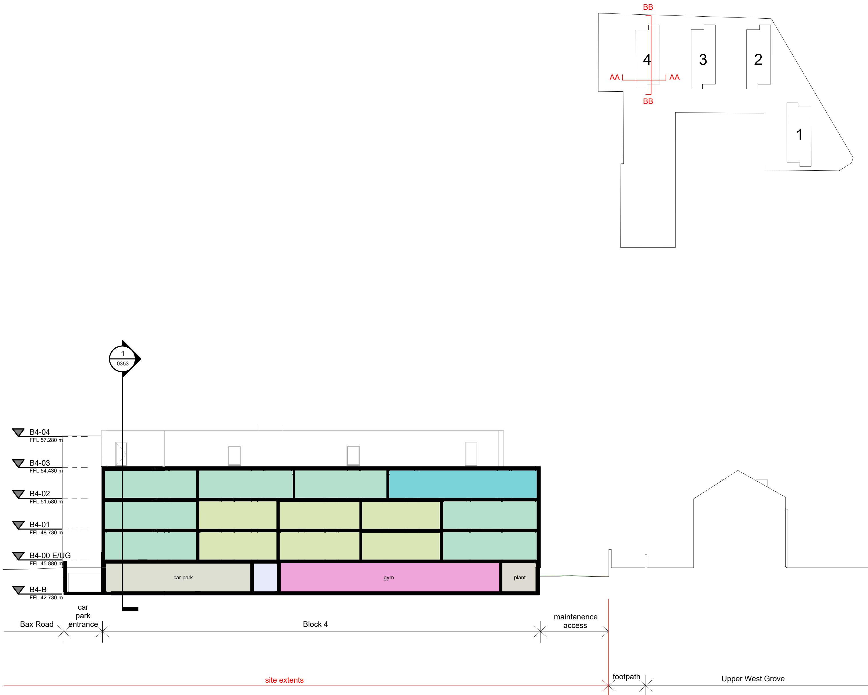
2 Existing Section BB 1 : 200
