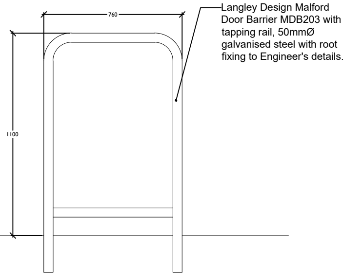
C6 Door Barrier - Section detail 1:20
